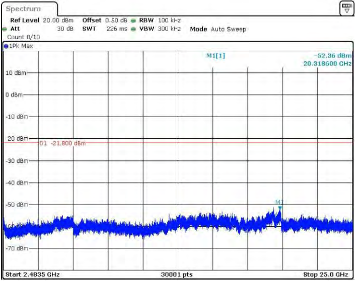
11GMINO_Ant2_2412_2483.5~25000
