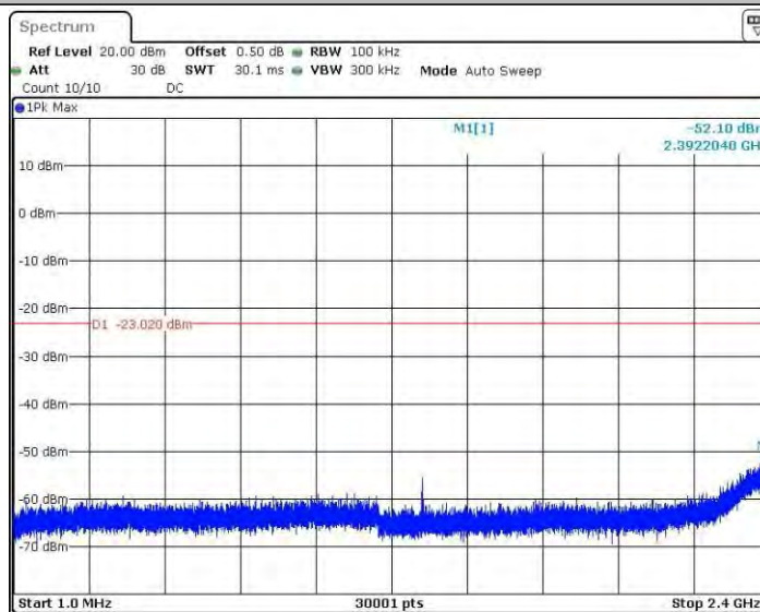
11B_Ant1_2462_0~Reference
