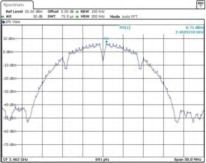
11B_Ant2_2462_0~Reference
