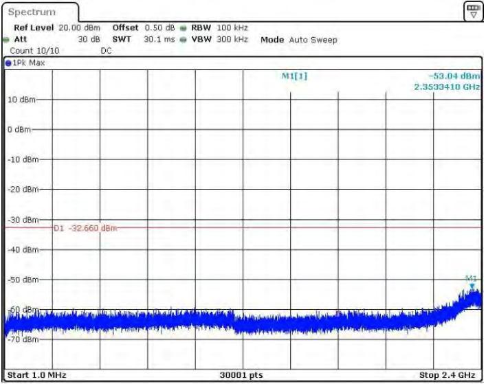
11N20SISO_Ant2_2462_1~2400
