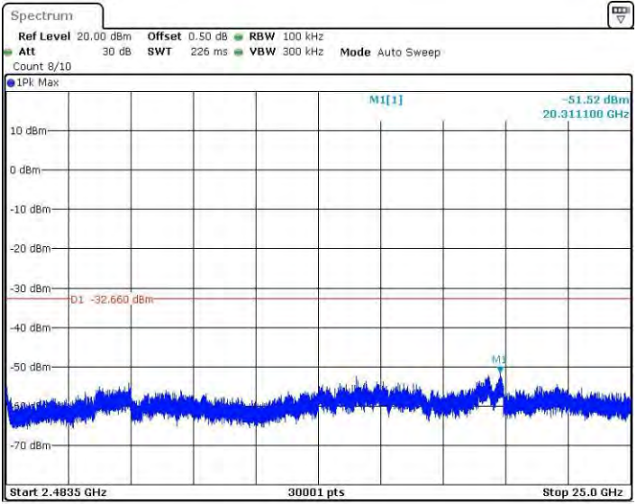
11N20SISO_Ant2_2462_2483.5~25000
