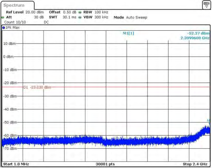
11B_Ant4_2462_1~2400
