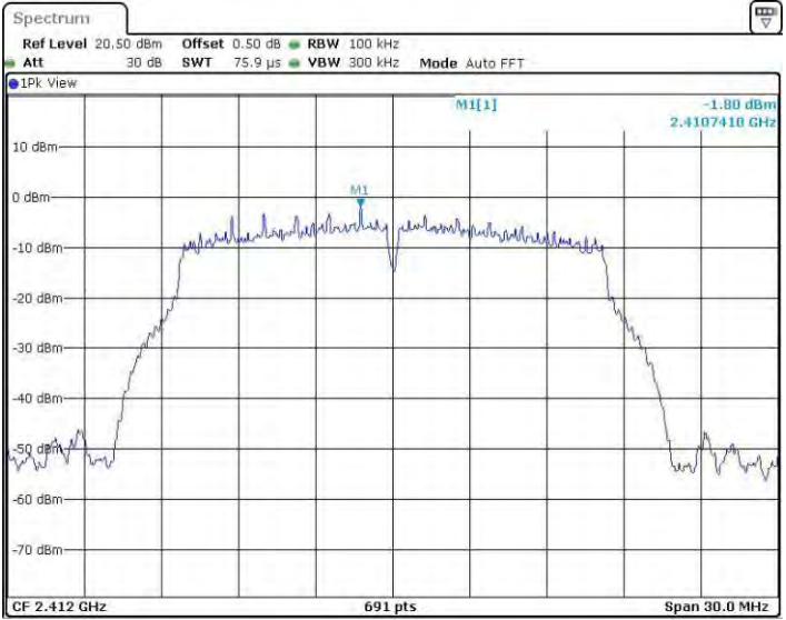
11GMINO_Ant2_2412_0-Reference
