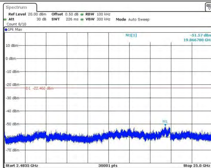
11GMINO_Ant2_2437_1~2400
