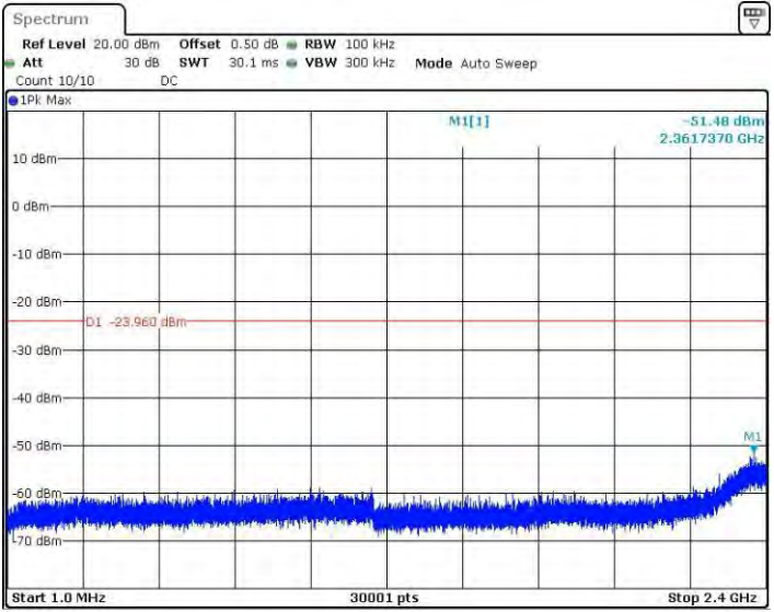
11B_Ant2_2437_1~2400
