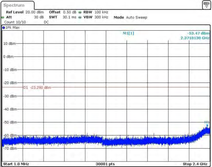
11B_Ant2_2462_1~2400
