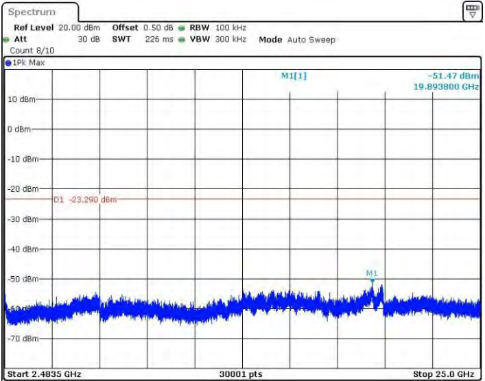
11B_Ant2_2462_2483.5~25000
