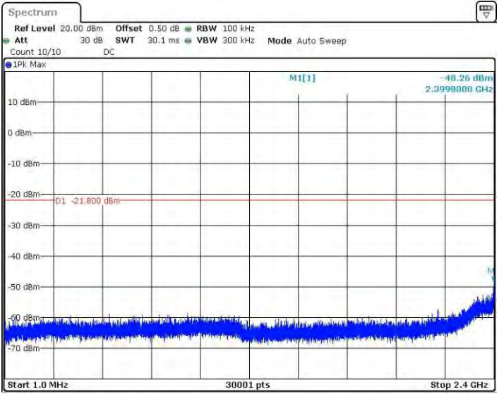
11GMINO_Ant2_2412_1~2400
