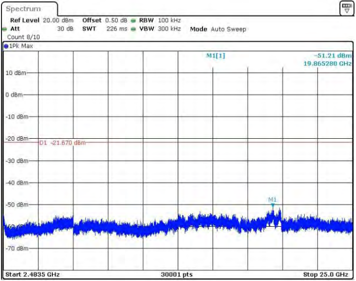
11GMINO_Ant3_2462_2483.5~25000
