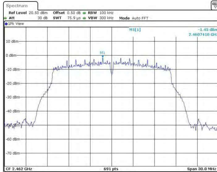
11GMINO_Ant2_2462_0-Reference
