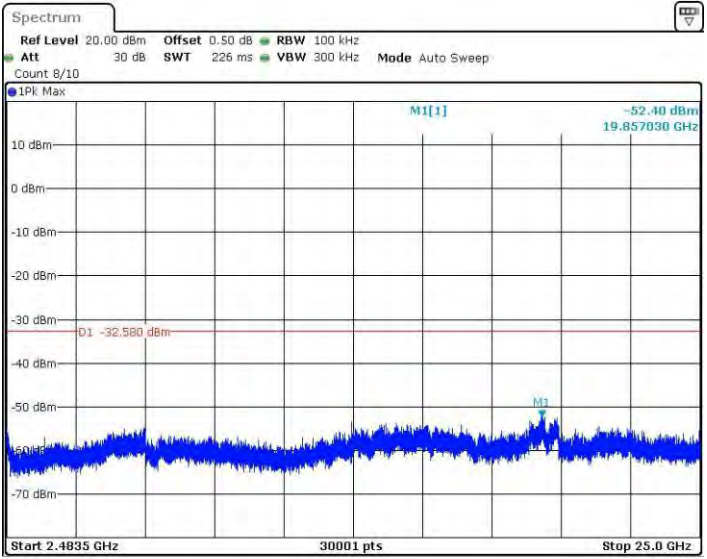
11N20SISO_Ant1_2462_2483.5~25000
