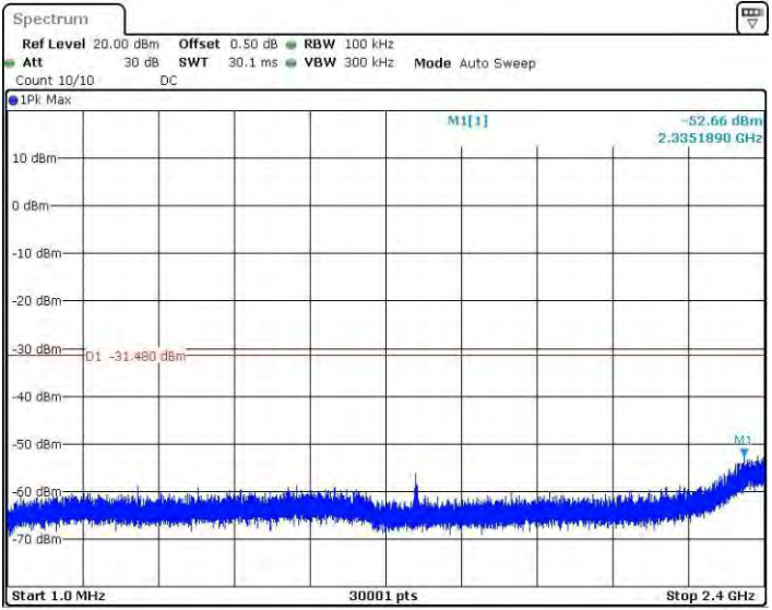
11G_Ant2_2462_1~2400
