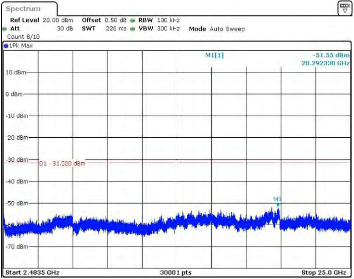
11G_Ant2_2412_2483.5~25000
