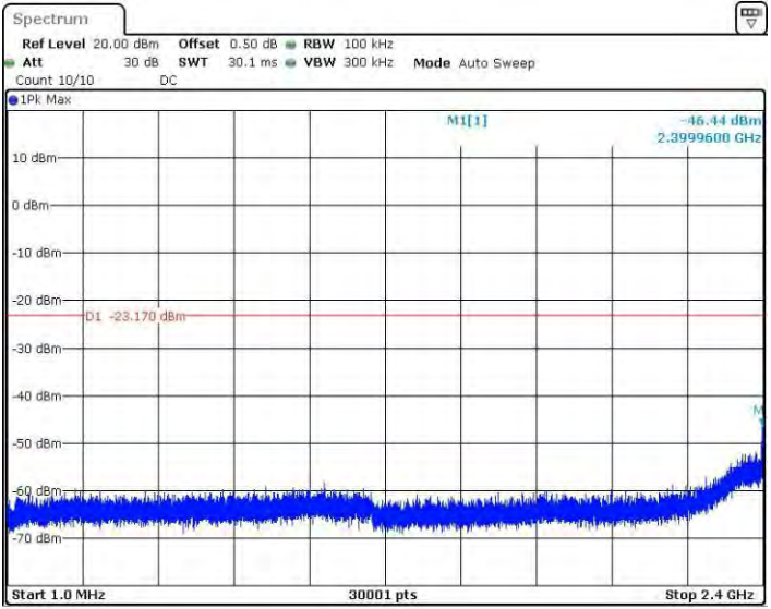
11B_Ant2_2412_1~2400
