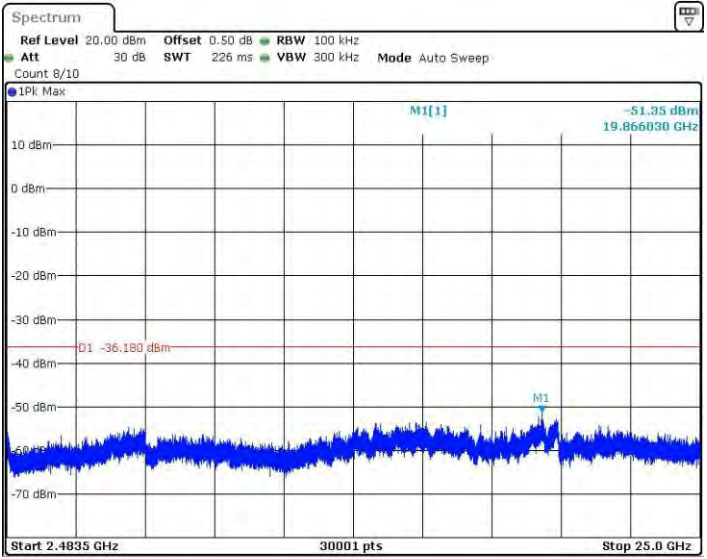
11N40SISO_Ant1_2422_2483.5~25000
