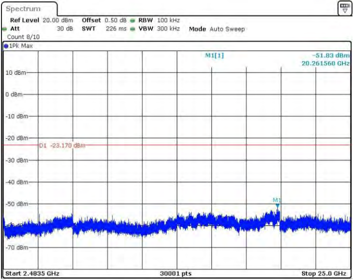
11B_Ant2_2412_2483.5~25000
