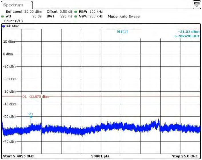
11N20SISO_Ant3_2462_2483.5~25000
