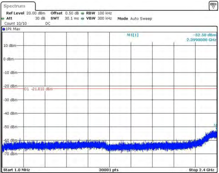
11GMINO_Ant4_2437_1~2400
