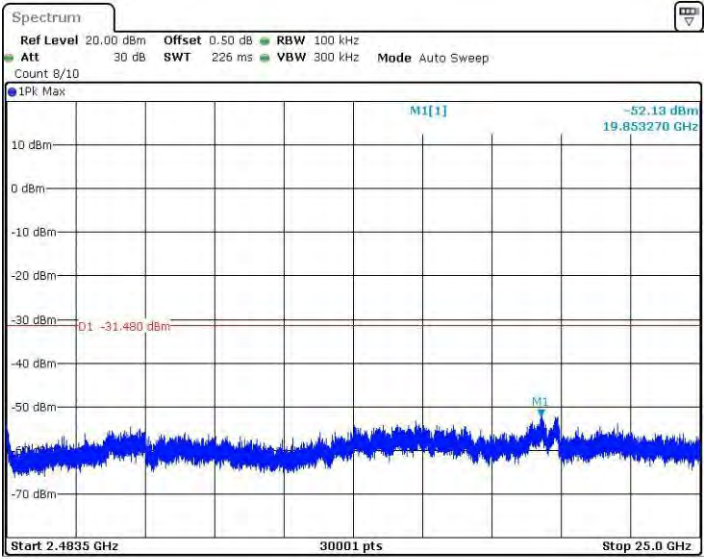
11G_Ant2_2462_2483.5~25000
