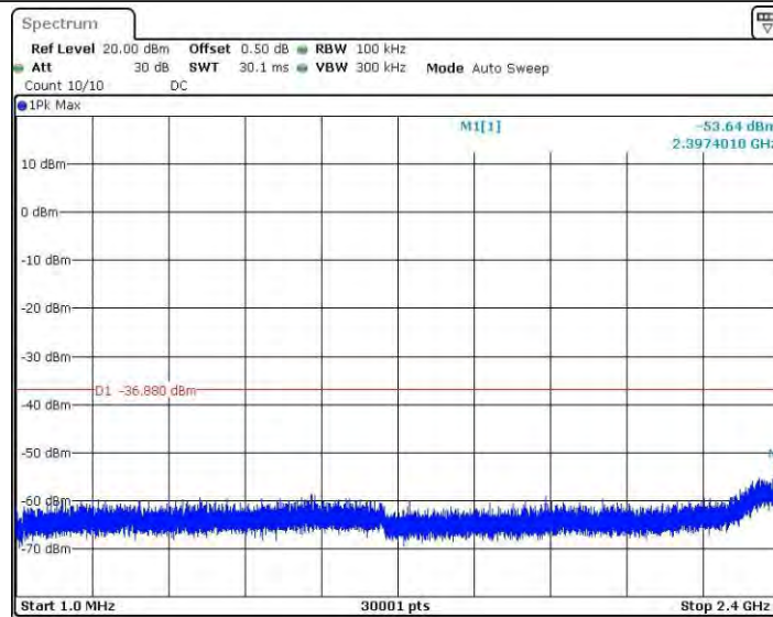
11N40SISO_Ant2_2437_1~2400
