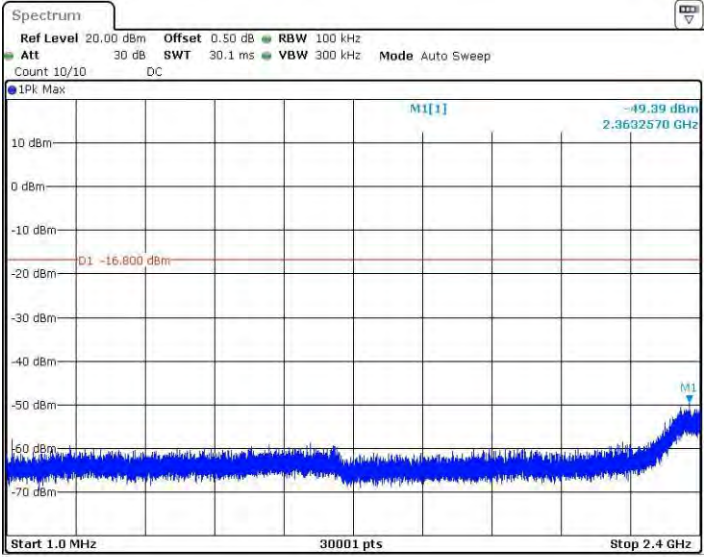
11N40SISO_Ant2_2452_1~2400
