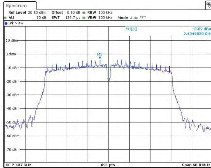
11N40MINO_Ant4_2437_0~Reference
