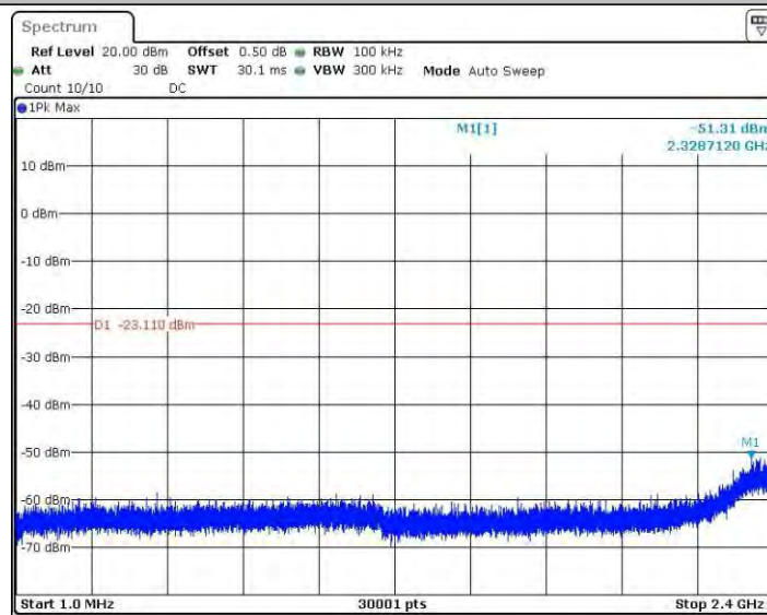
11N40MINO_Ant3_2452_0~Reference
