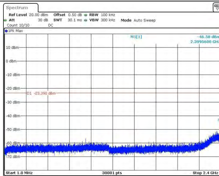
11N40MINO_Ant4_2422_0~Reference
