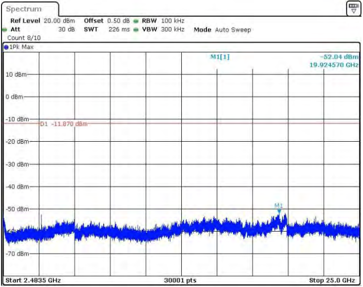
11BMINO_Ant1_2437_2483.5~25000
