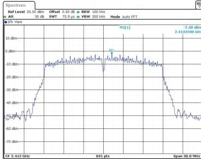
11N20MINO_Ant3_2412_0~Reference
