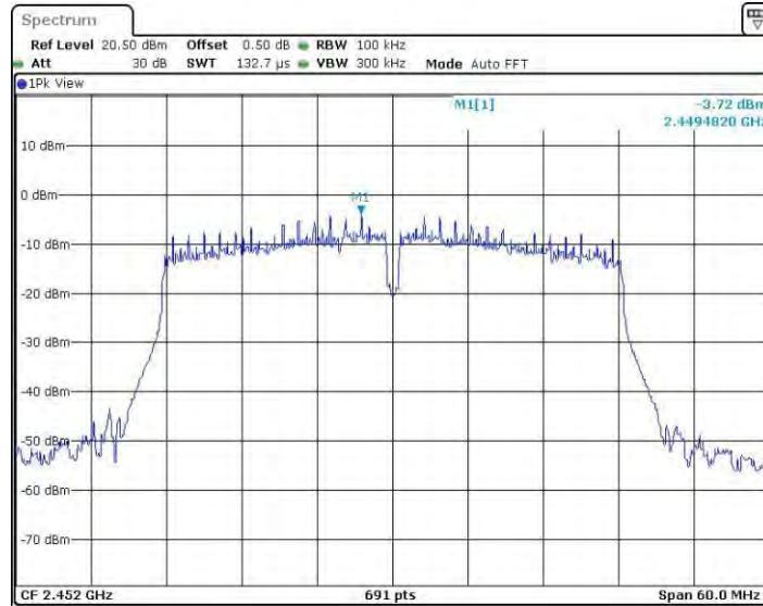
11N40MINO_Ant2_2452_0~Reference
