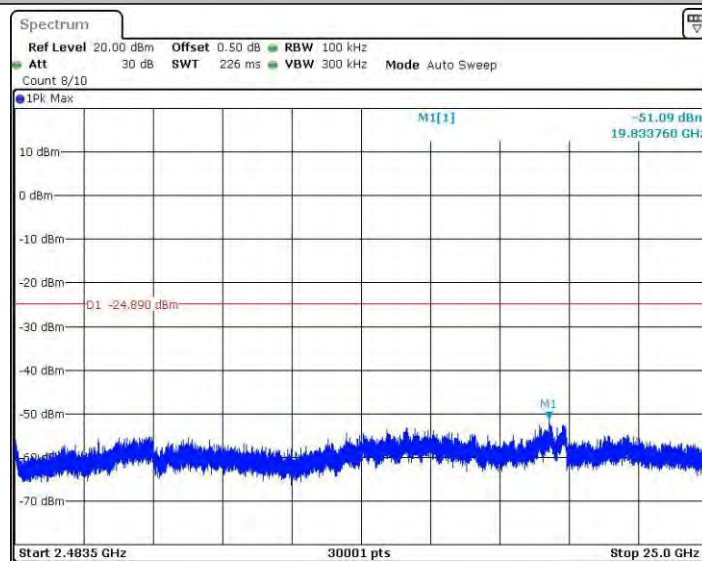
11N40MINO_Ant2_2437_2483.5~25000
