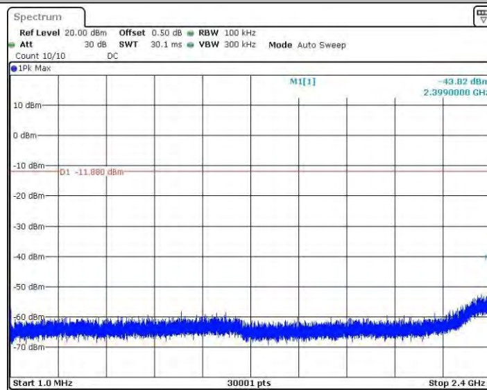
11BMINO_Ant2_2412_0~Reference
