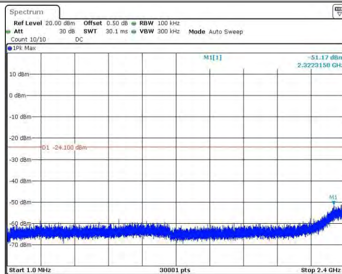
11N40MINO_Ant3_2437_0~Reference
