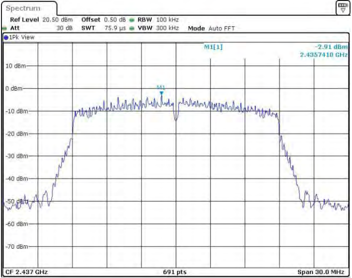
11N20MINO_Ant3_2437_0~Reference
