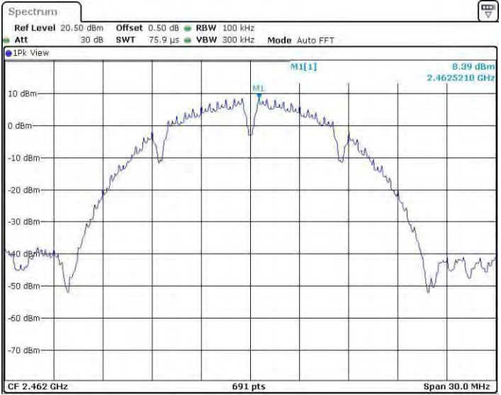
11BMINO_Ant2_2462_0~Reference
