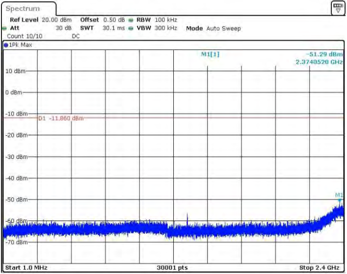
11BMINO_Ant1_2462_1~2400
