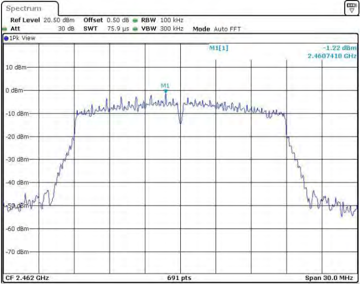
11N20MINO_Ant2_2462_0~Reference
