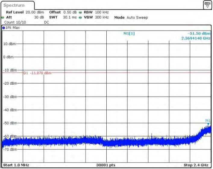
11BMINO_Ant1_2437_1~2400
