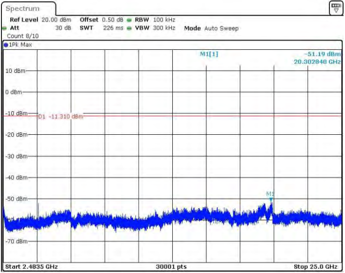
11BMINO_Ant1_2412_2483.5~25000
