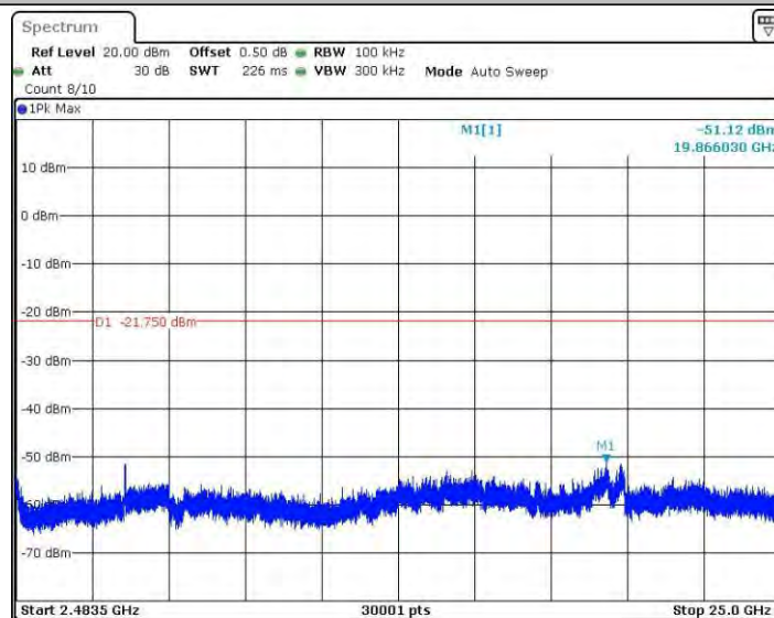
11N20MINO_Ant1_2412_2483.5~25000
