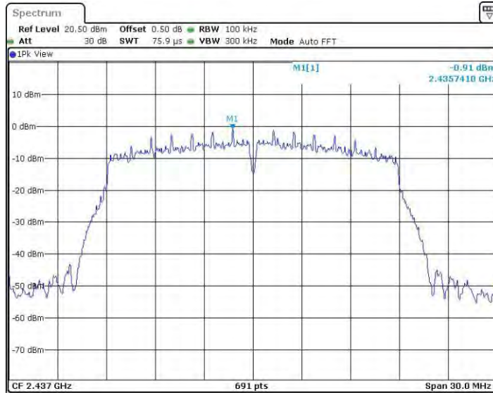
11N20MINO_Ant4_2437_0~Reference
