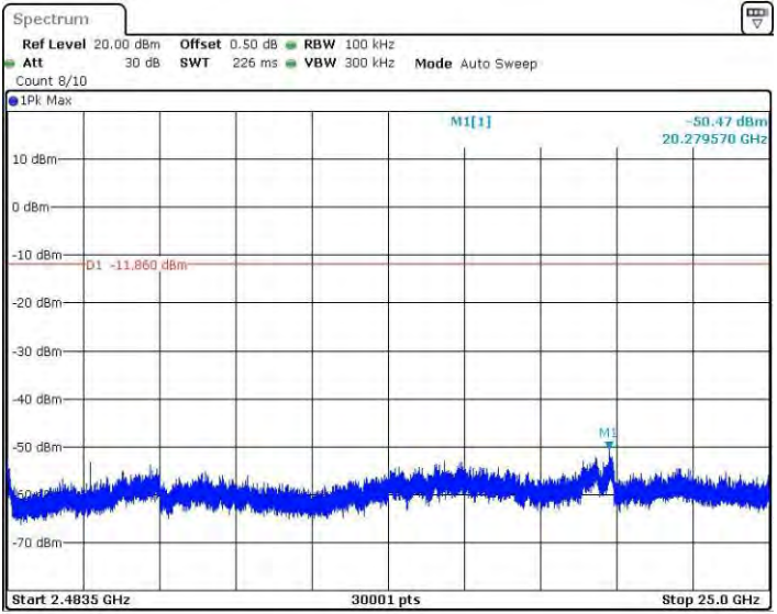
11BMINO_Ant1_2462_2483.5~25000
