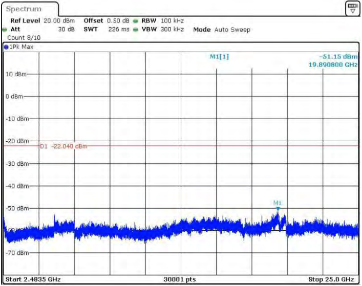
11N20MINO_Ant1_2437_2483.5~25000
