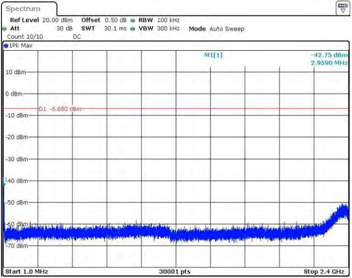
11BSISO_Ant2_2462_1~2400
