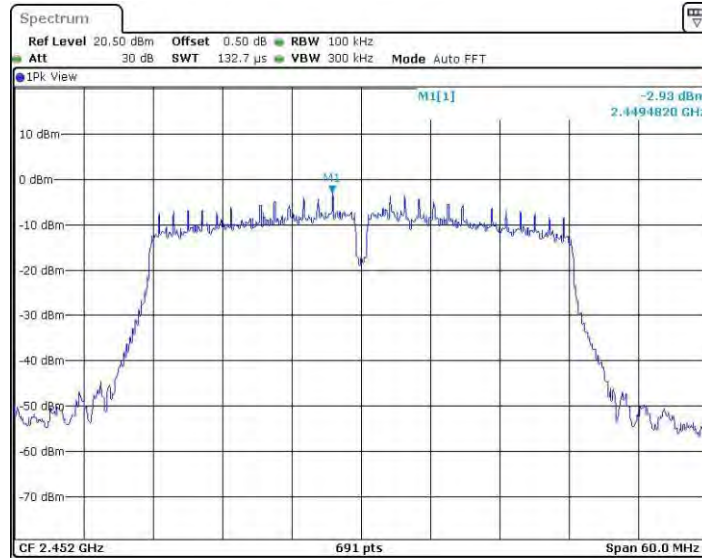
11N40MINO_Ant4_2452_0~Reference
