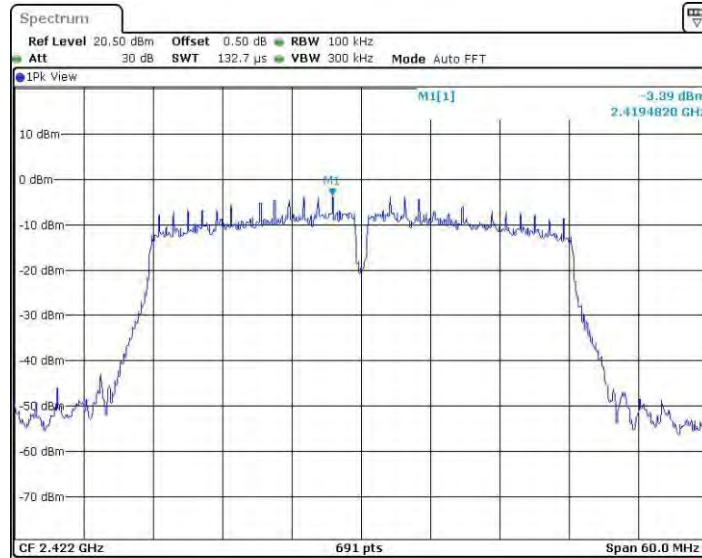
11N40MINO_Ant4_2422_0~Reference
