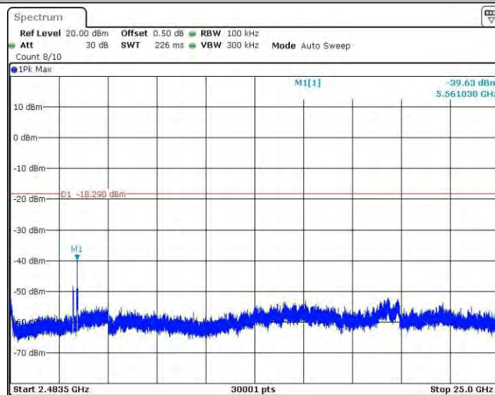
11N40SISO_Ant3_2422_2483.5~25000
