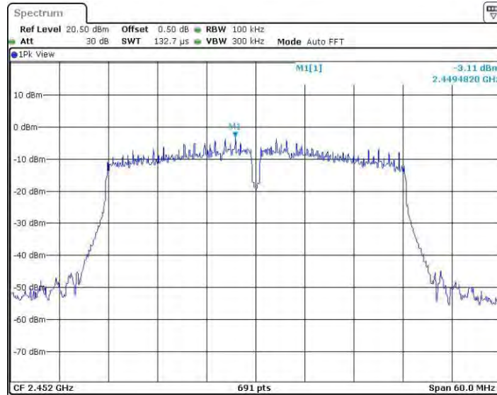
11N40MINO_Ant3_2452_0~Reference
