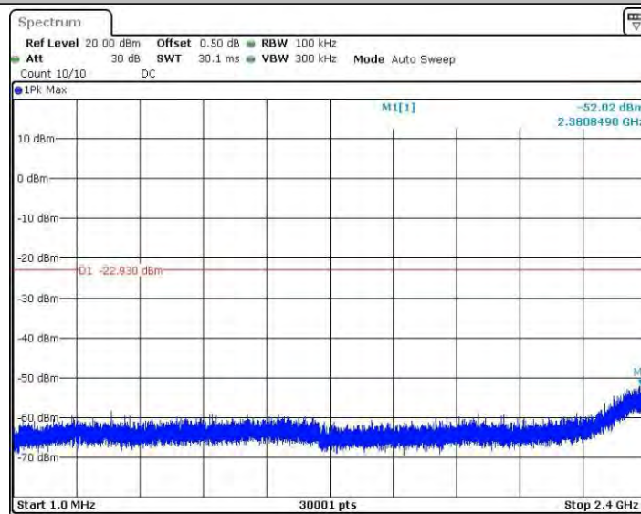
11N40MINO_Ant4_2452_0~Reference
