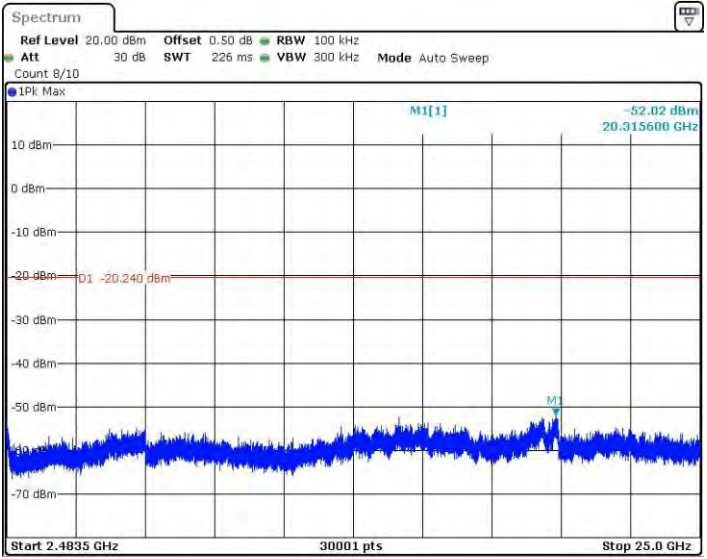
11N20MINO_Ant4_2412_2483.5~25000
