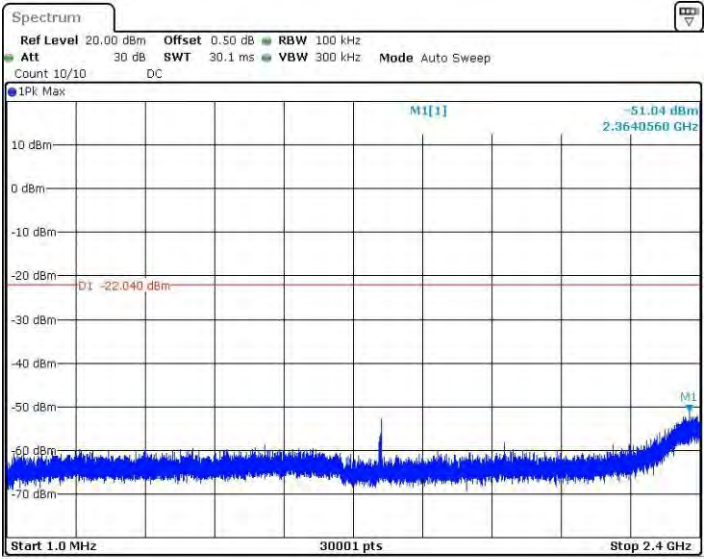
11N20MINO_Ant1_2437_1~2400
