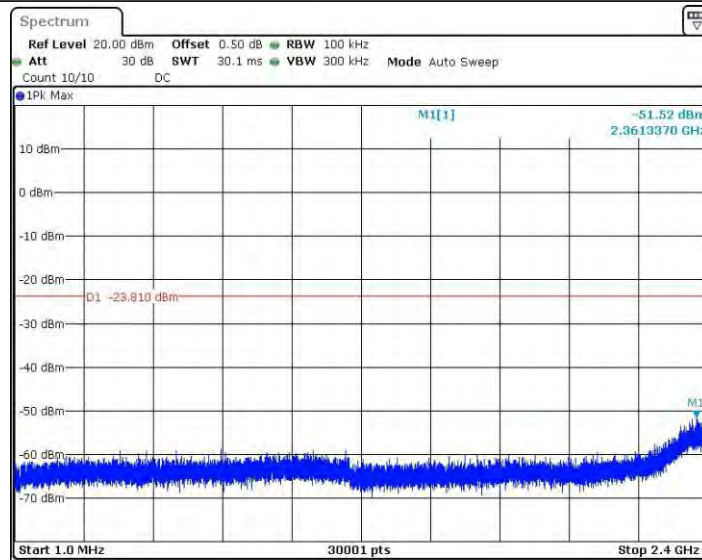
11N40MINO_Ant1_2437_1~2400
