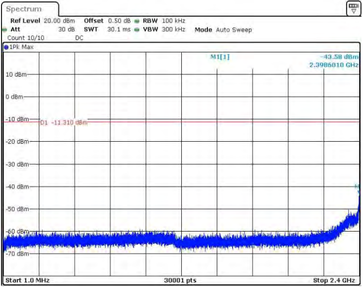
11BMINO_Ant1_2412_1~2400
