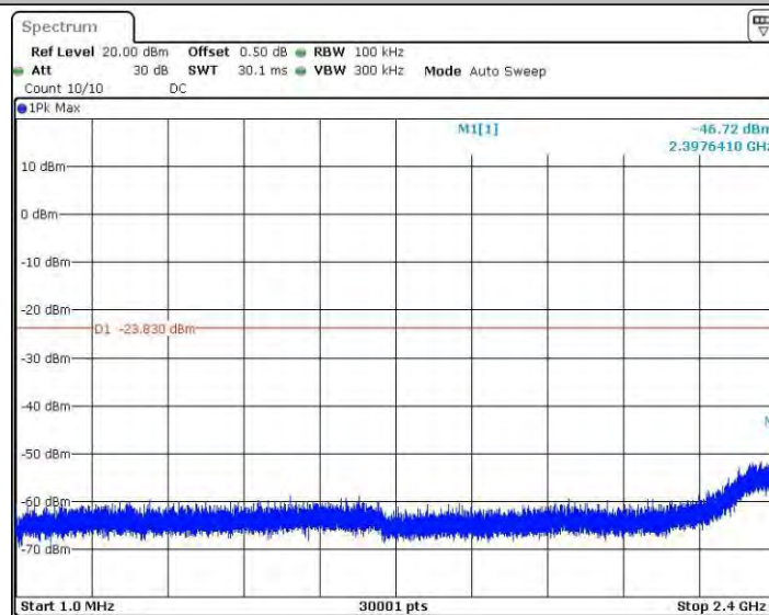
11N40MINO_Ant3_2422_0~Reference
