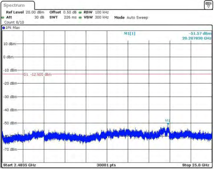
11BMINO_Ant3_2437_2483.5~25000
