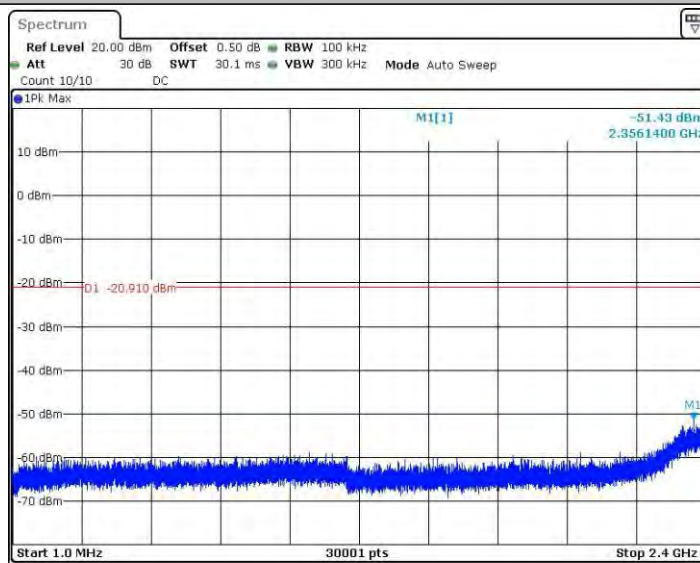
11N20MINO_Ant4_2437_0~Reference
