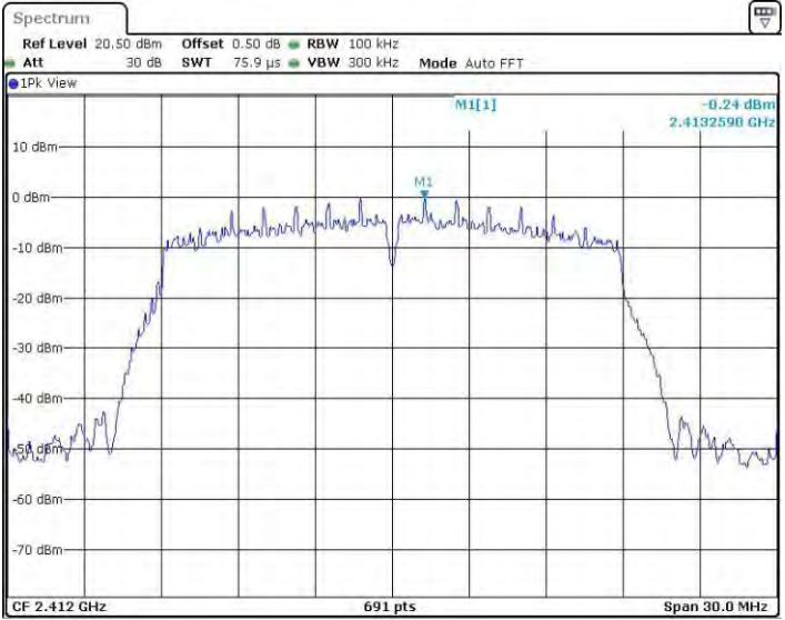
11N20MINO_Ant4_2412_0~Reference
