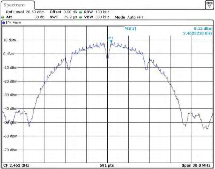
11BMINO_Ant3_2462_0~Reference
