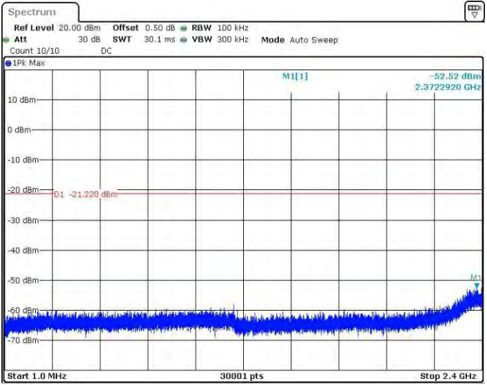
11N20MINO_Ant2_2462_1~2400
