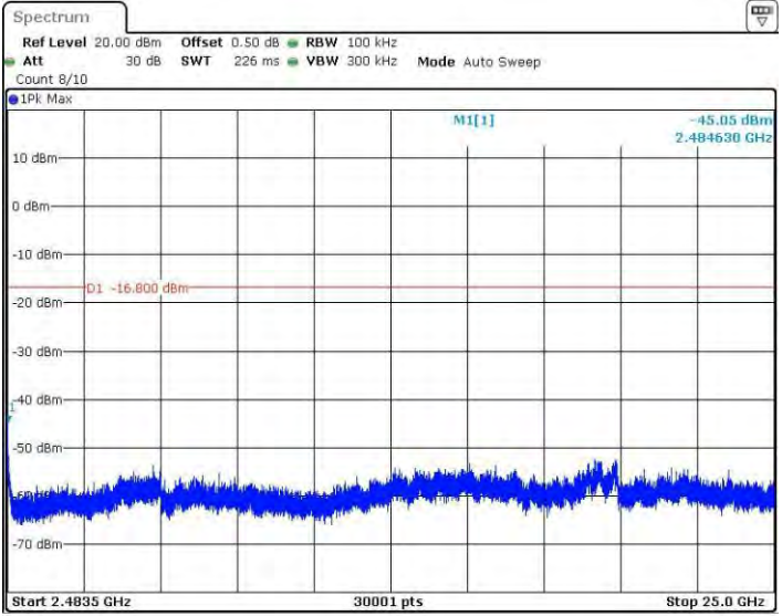
11N40SISO_Ant2_2452_2483.5~25000
