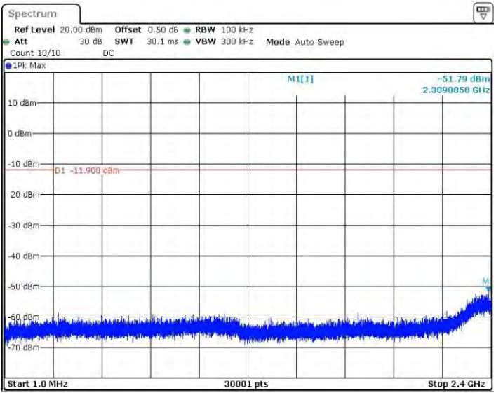
11BMINO_Ant4_2437_1~2400
