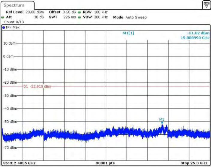
11N20MINO_Ant3_2437_2483.5~25000
