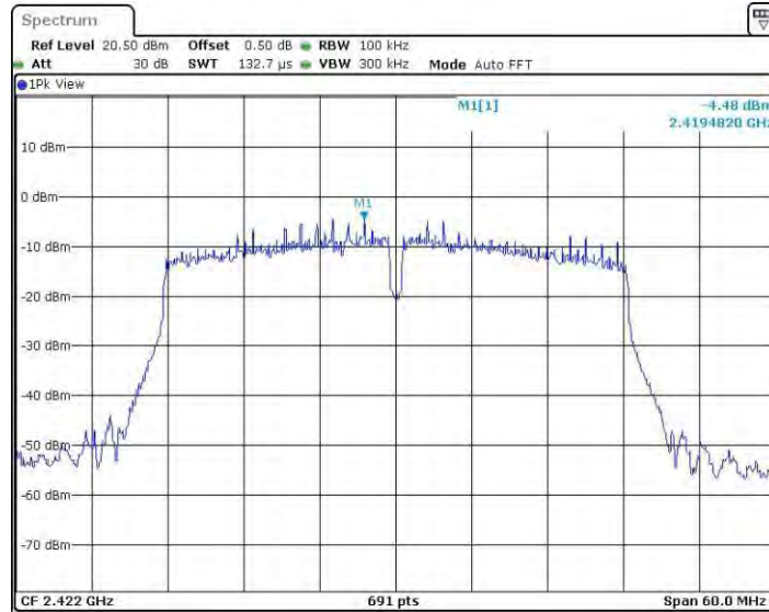
11N40MINO_Ant2_2422_0~Reference
