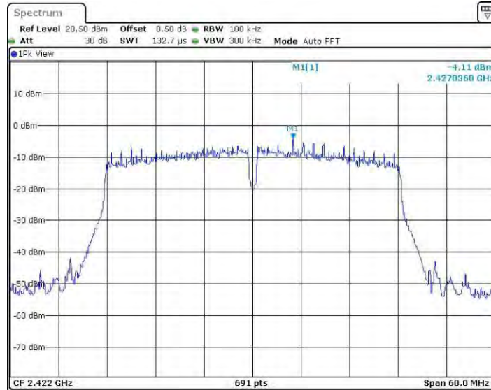
11N40MINO_Ant1_2422_0~Reference
