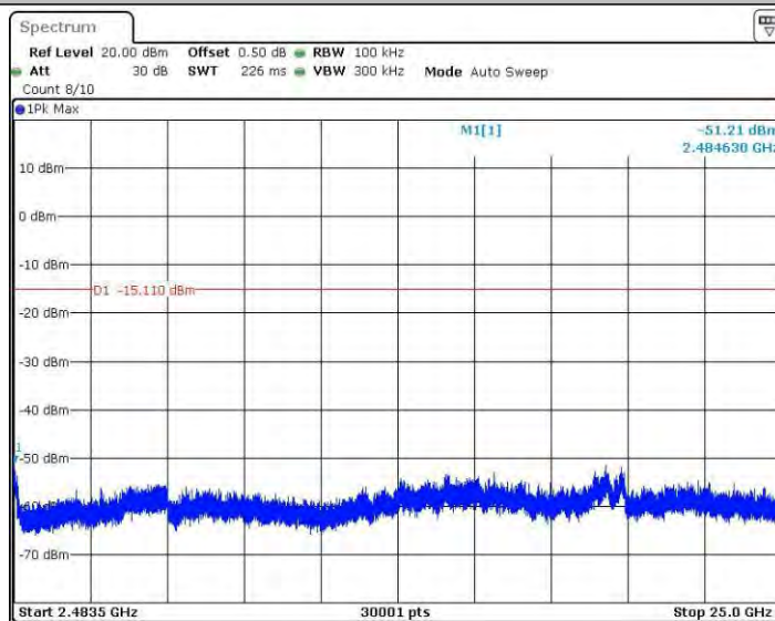
11N20SISO_Ant3_2462_2483.5~25000
