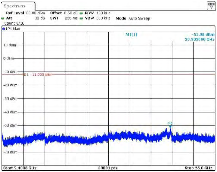
11BMINO_Ant4_2437_2483.5~25000
