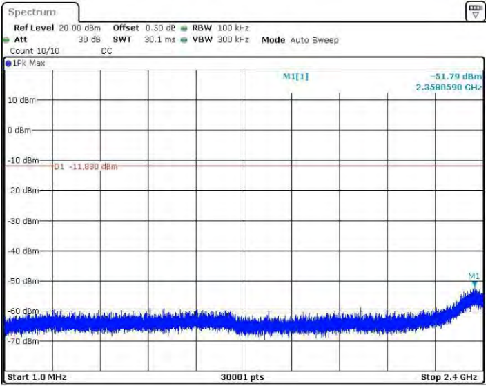
11BMINO_Ant3_2462_1~2400
