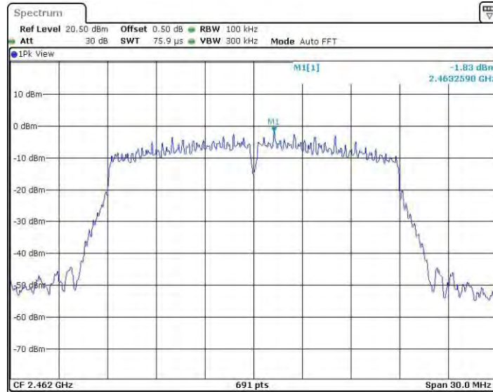
11N20MINO_Ant3_2462_0~Reference
