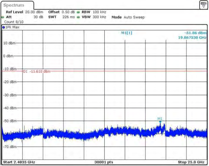
11BMINO_Ant2_2462_2483.5~25000
