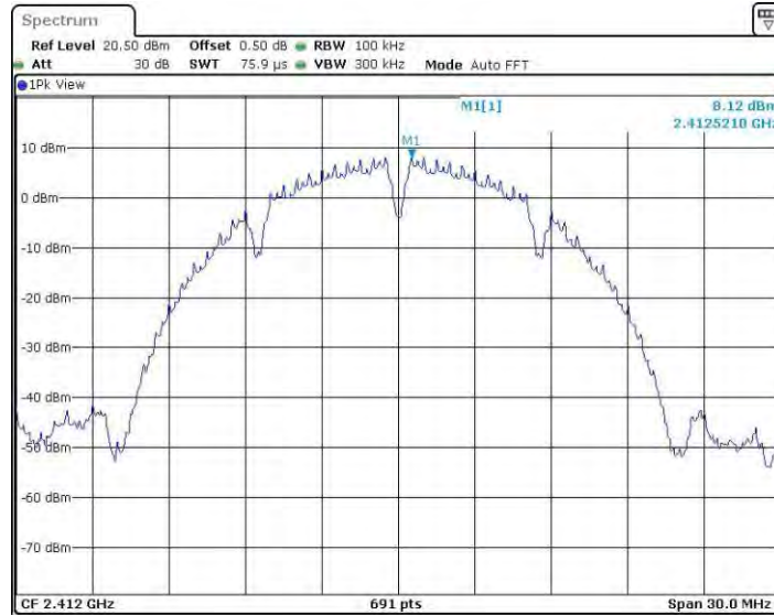
11BMINO_Ant2_2412_0~Reference
