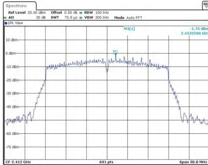
11N20MINO_Ant1_2412_0~Reference
