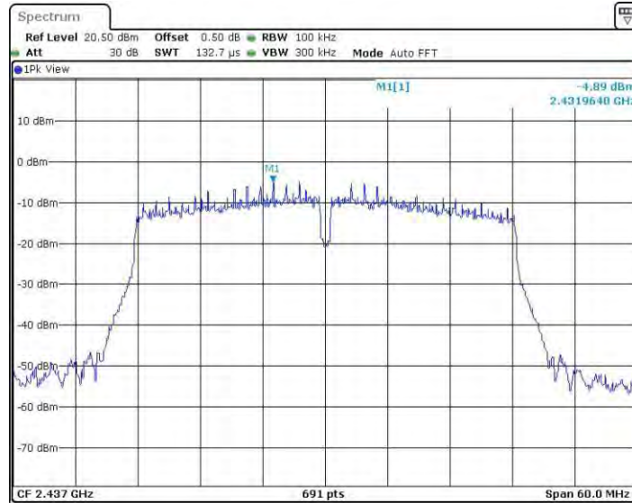
11N40MINO_Ant2_2437_0~Reference
