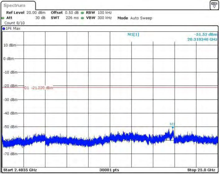
11N20MINO_Ant2_2462_2483.5~25000
