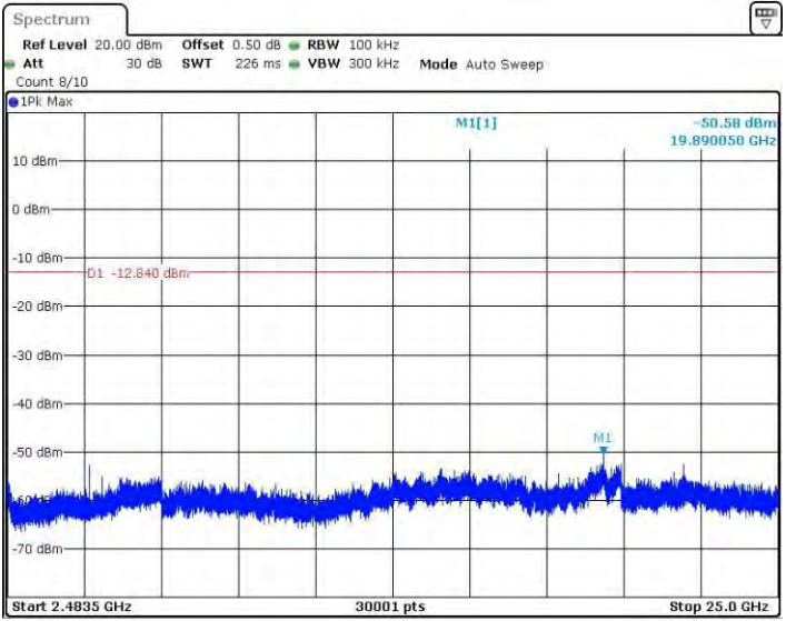
11BMINO_Ant2_2437_2483.5~25000
