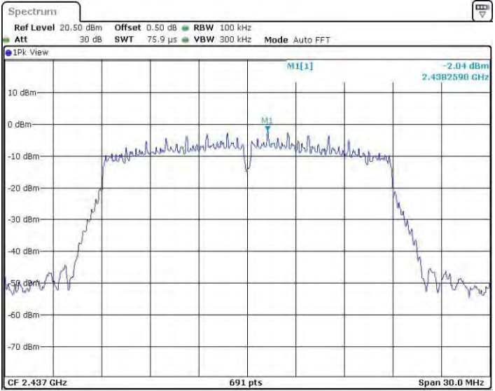
11N20MINO_Ant1_2437_0~Reference
