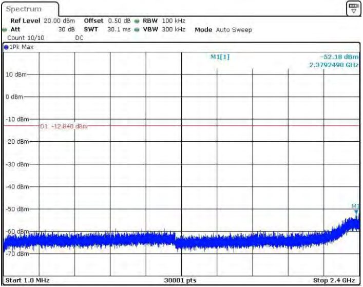
11BMINO_Ant2_2437_1~2400
