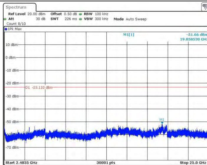
11N40MINO_Ant3_2452_1~2400
