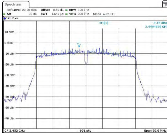
11N40MINO_Ant1_2452_0~Reference
