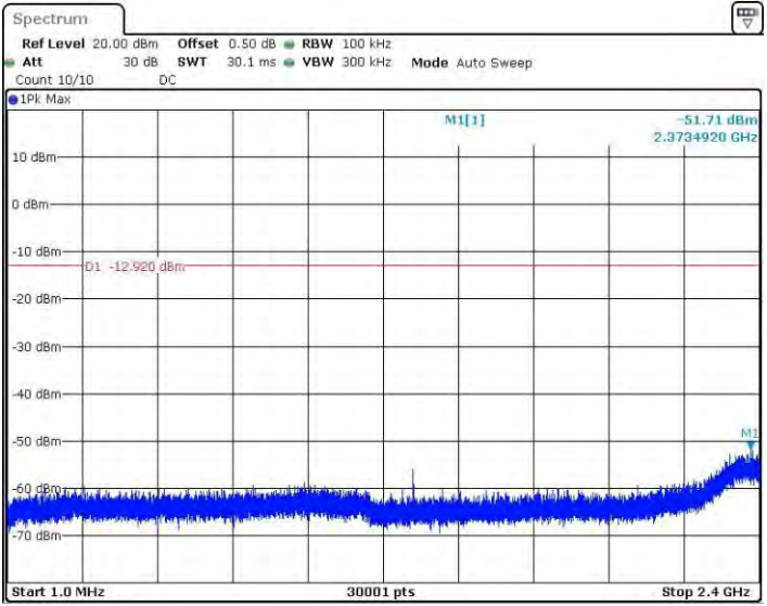
11BMINO_Ant3_2437_1~2400
