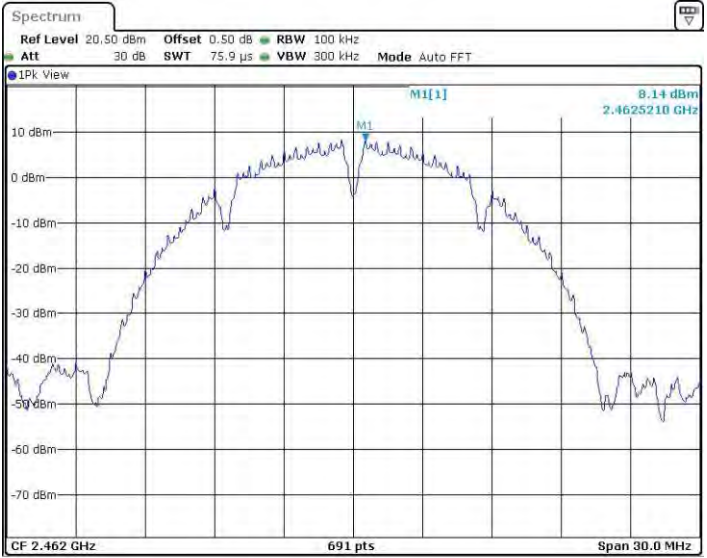
11BMINO_Ant1_2462_0~Reference
