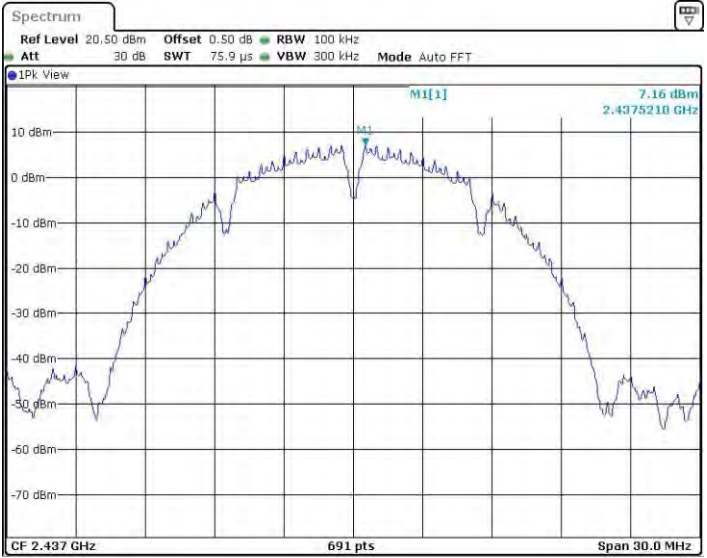
11BMINO_Ant2_2437_0~Reference
