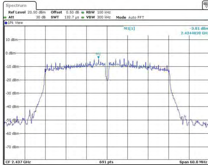
11N40MINO_Ant1_2437_0~Reference
