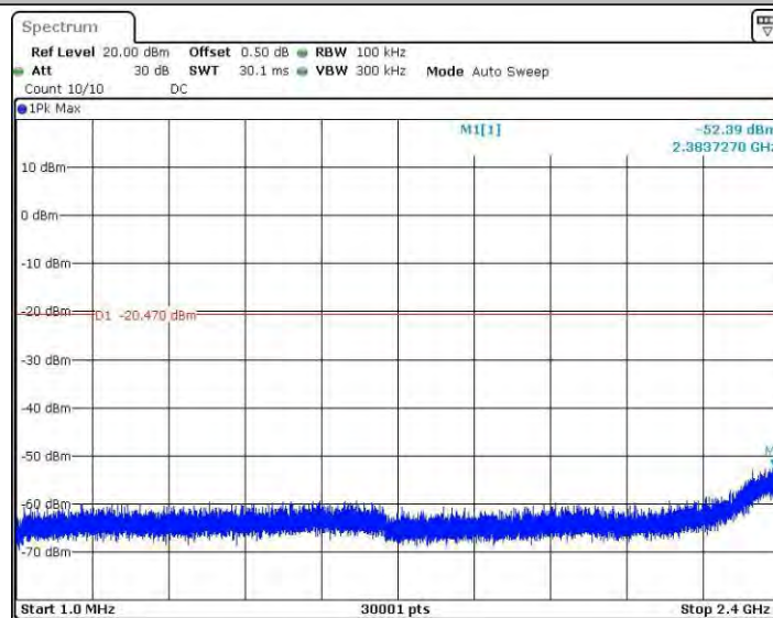
11N20MINO_Ant4_2462_0~Reference
