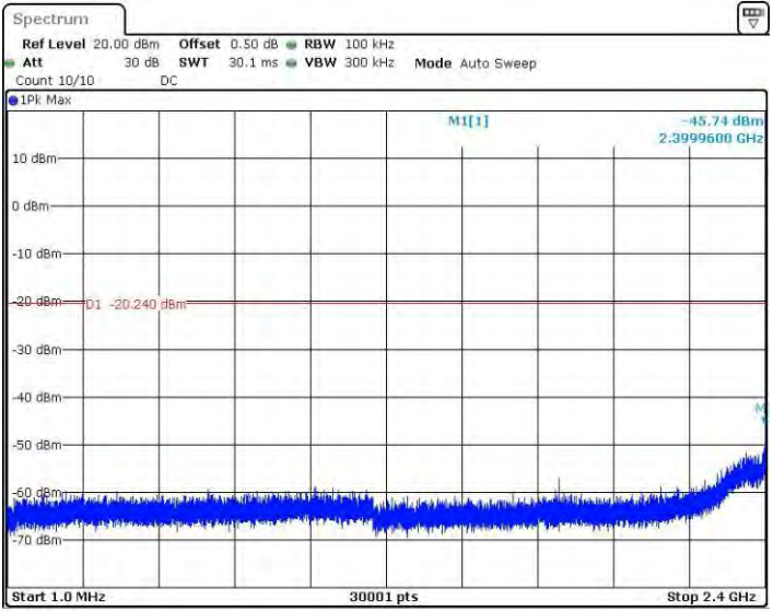
11N20MINO_Ant4_2412_1~2400
