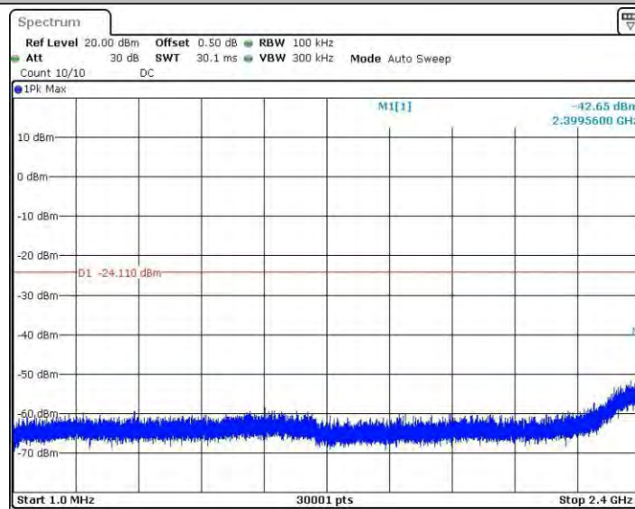
11N40MINO_Ant1_2422_0~Reference
