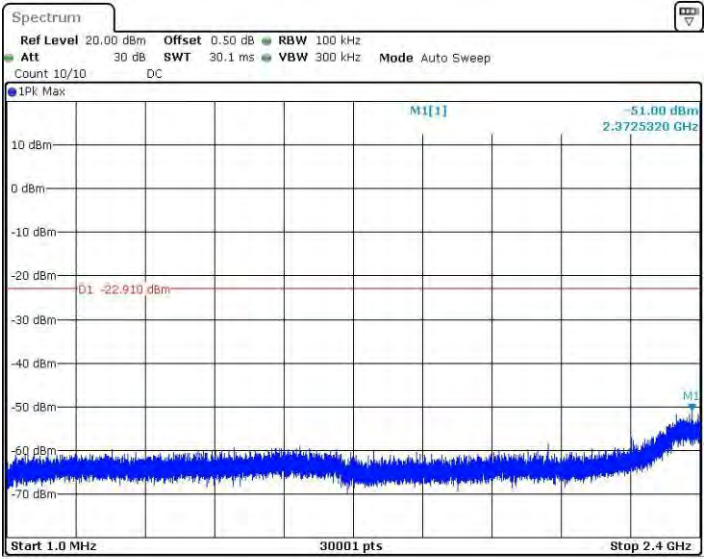
11N20MINO_Ant3_2437_1~2400
