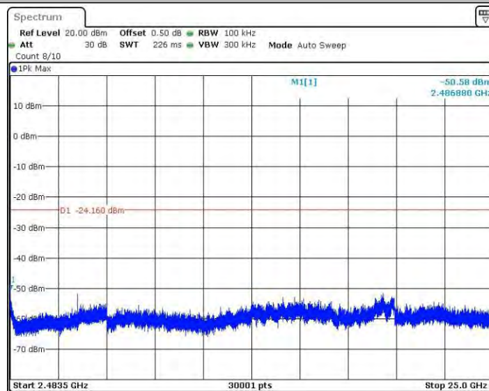
11N40MINO_Ant1_2452_1~2400
