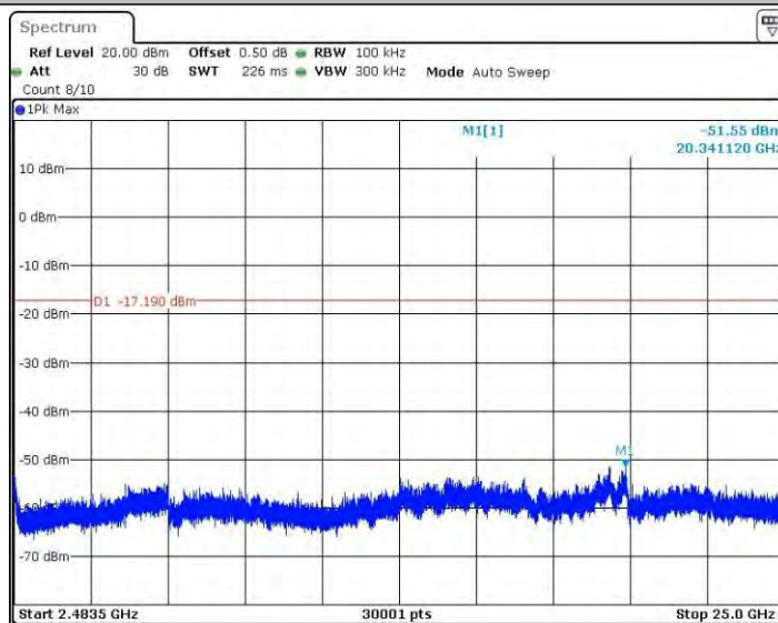
11N40SISO_Ant2_2422_1~2400
