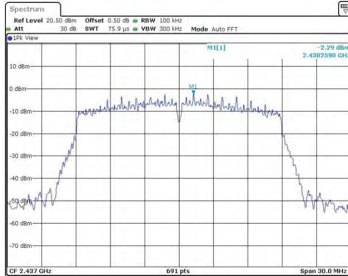
11N20MINO_Ant2_2437_0~Reference
