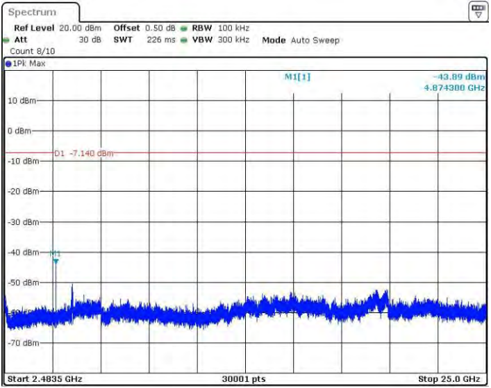
11BSISO_Ant2_2437_2483.5~25000
