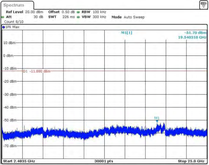
11BMINO_Ant3_2462_2483.5~25000
