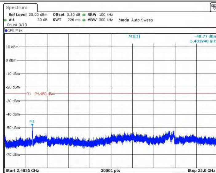
11N40MINO_Ant2_2422_2483.5~25000
