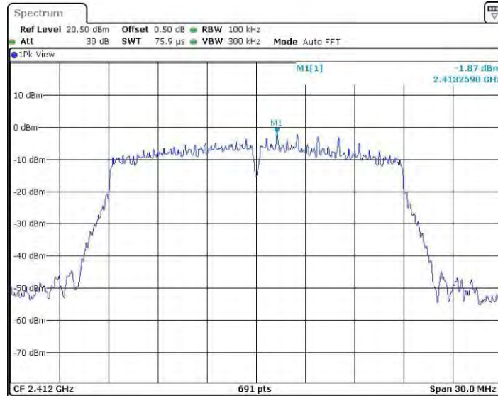
11N20MINO_Ant2_2412_0~Reference
