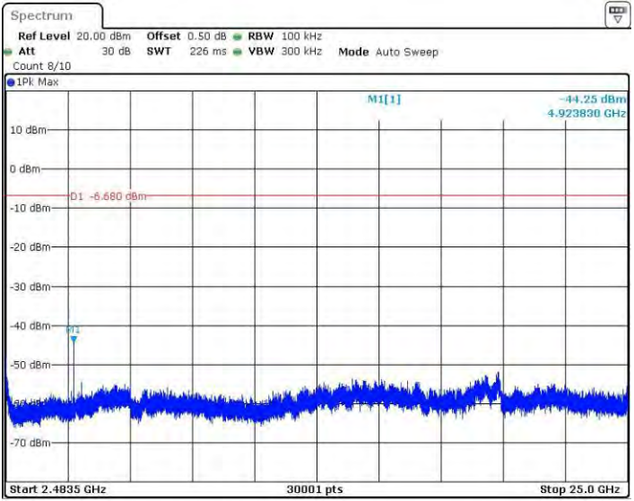
11BSISO_Ant2_2462_2483.5~25000
