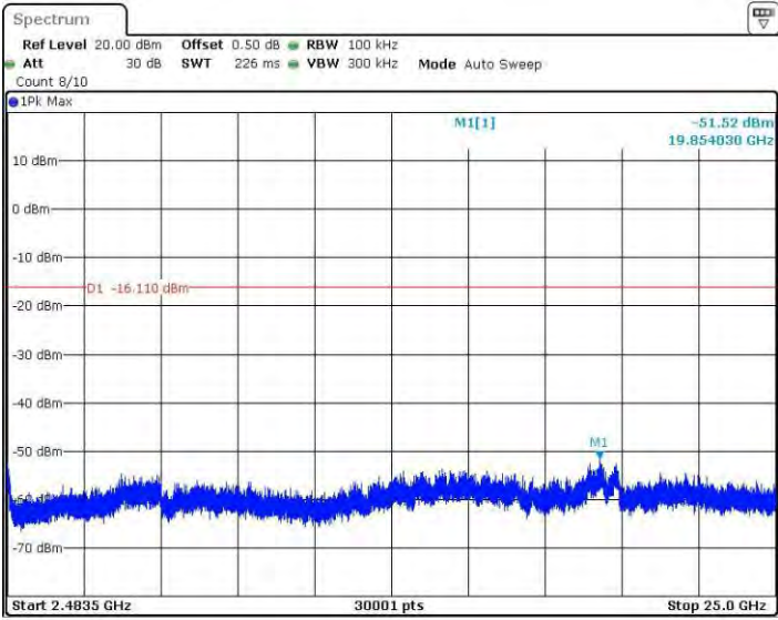
11GSISO_Ant2_2437_2483.5~25000
