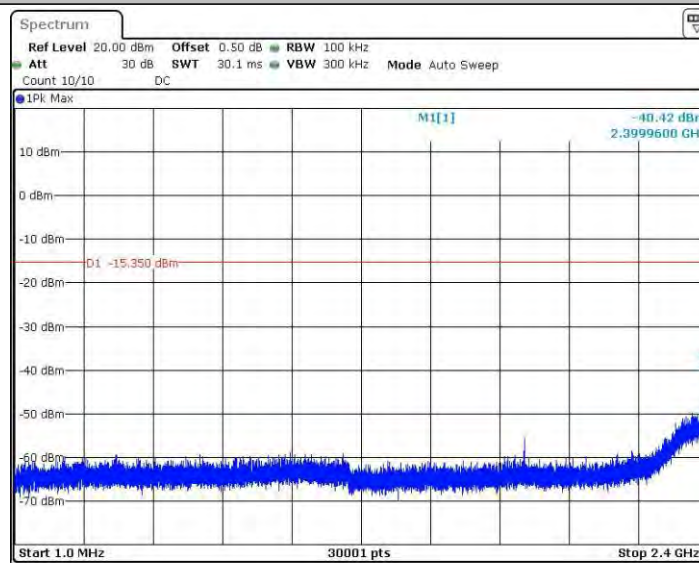
11GSISO_Ant2_2412_0~Reference
