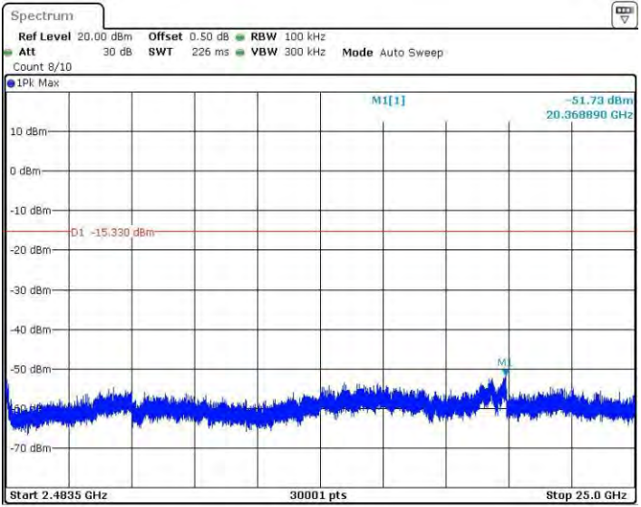
11GSISO_Ant1_2437_2483.5~25000
