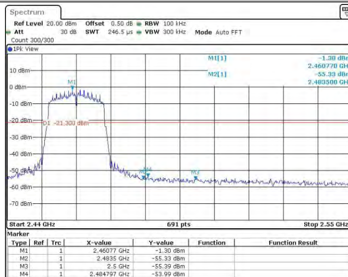
11N20MINO_Ant1_High_2462
