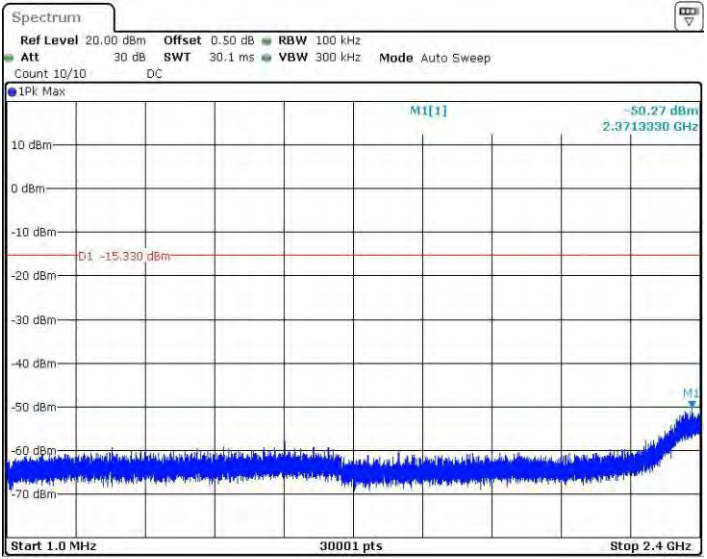
11GSISO_Ant1_2437_1~2400
