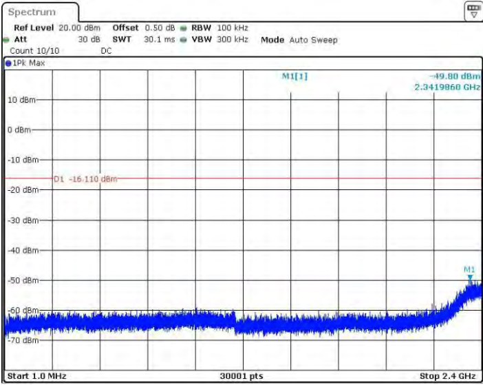
11GSISO_Ant2_2437_1~2400
