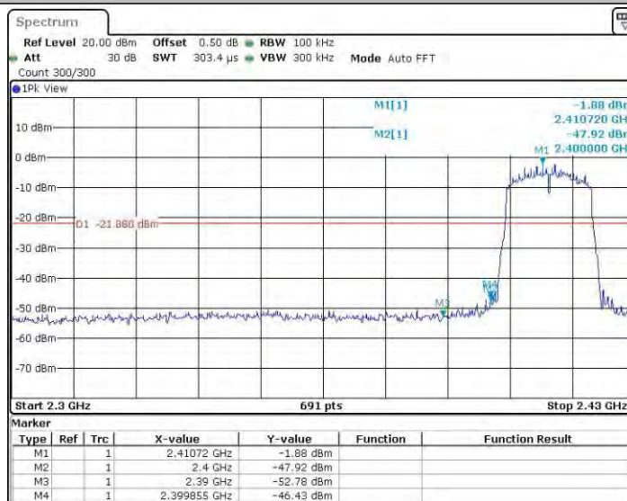
11N20MINO_Ant2_Low_2412
