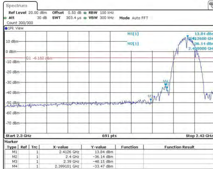
11BSISO_Ant1_Low_2412
