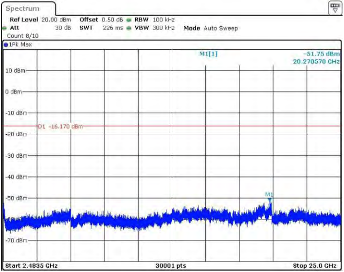
11N20SISO_Ant2_2437_2483.5~25000
