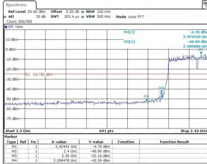
11N40MINO_Ant2_Low_2422
