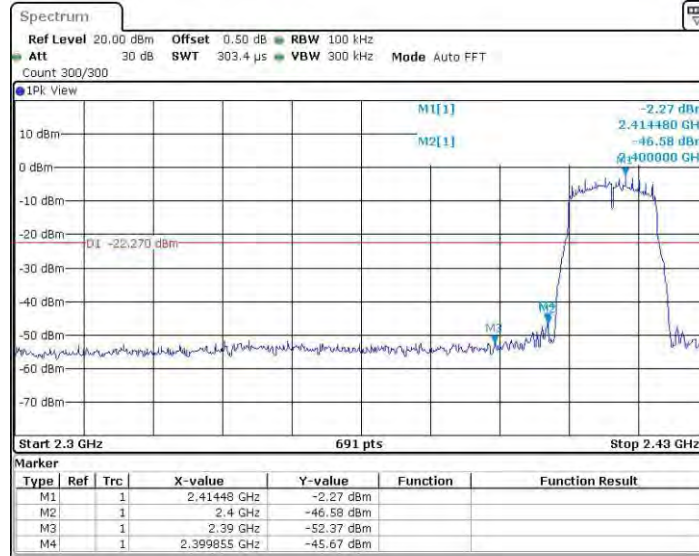
11GMINO_Ant2_Low_2412
