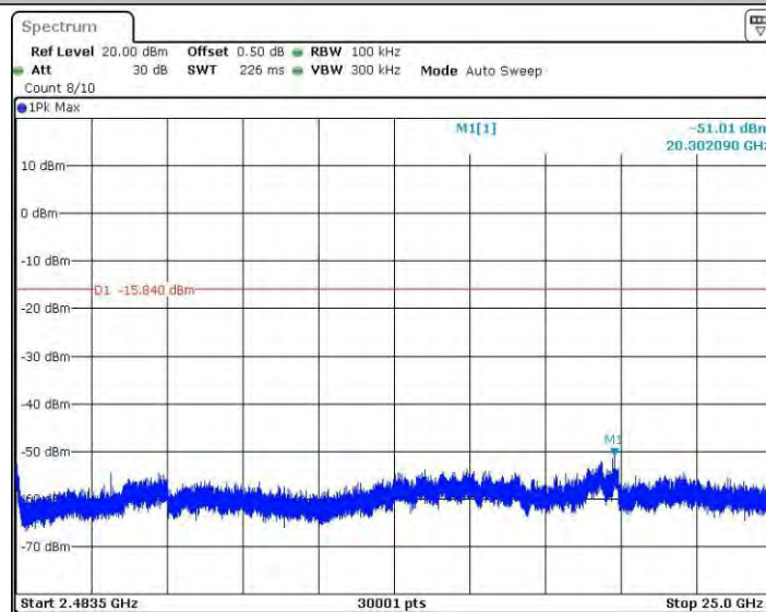
11GSISO_Ant4_2437_2483.5~25000
