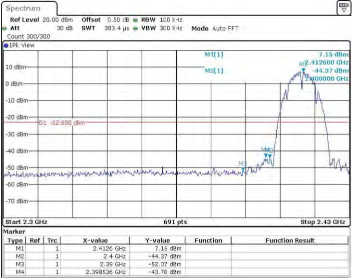
11B_Ant4_Low_2412
