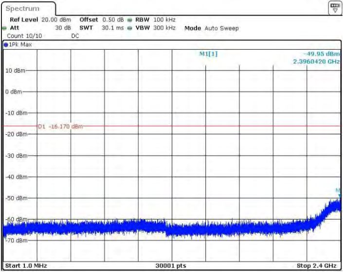
11N20SISO_Ant2_2437_1~2400
