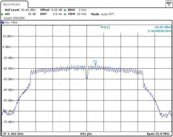
11GSISO_Ant4_2462
