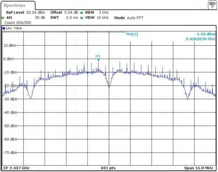
11BSISO_Ant2_2437
