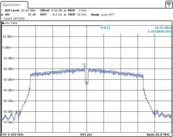
11N40MIMO_Ant3_2422
