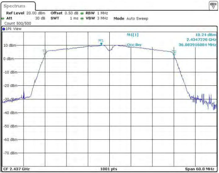
11N40SISO_Ant4_2437
