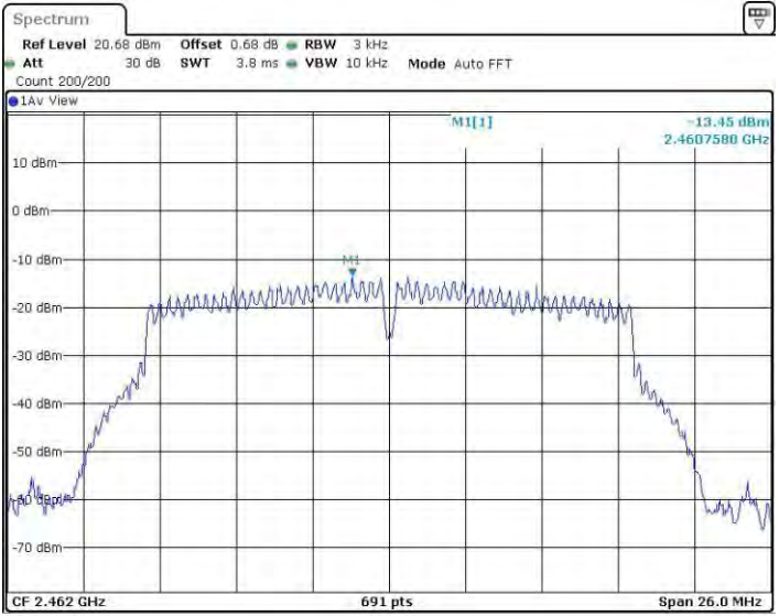
11G MIMO_Ant3_2462
