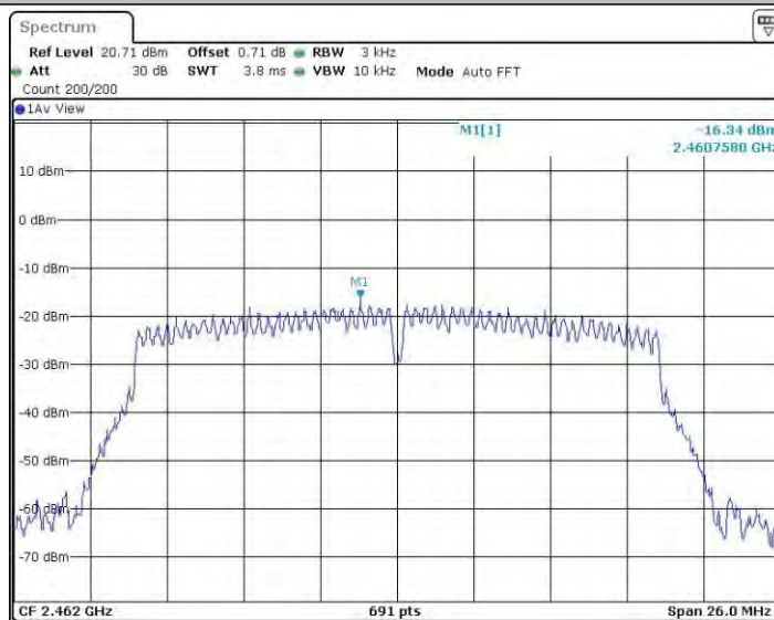
11N20SISO_Ant3_2462
