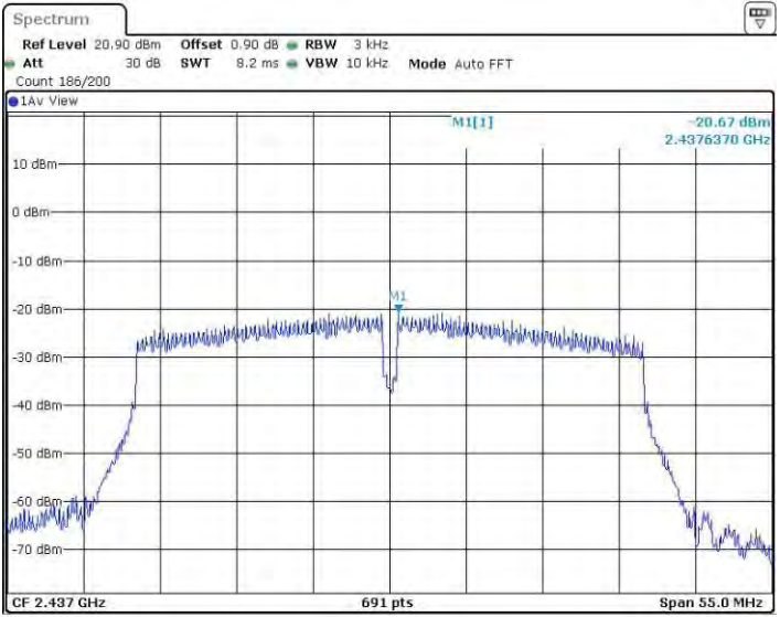
11N40SISO_Ant2_2437
