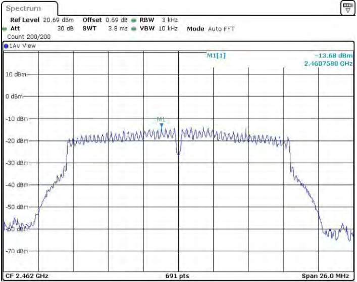
11G MIMO_Ant2_2462
