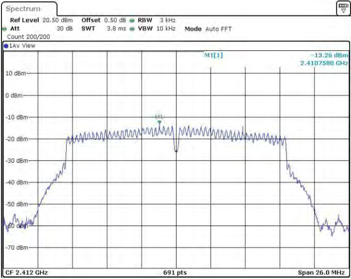
11G MIMO_Ant2_2412
