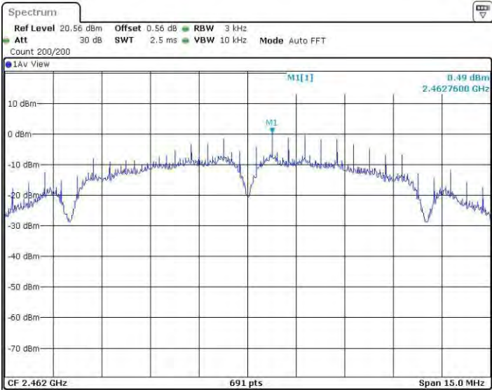
11BSISO_Ant1_2462
