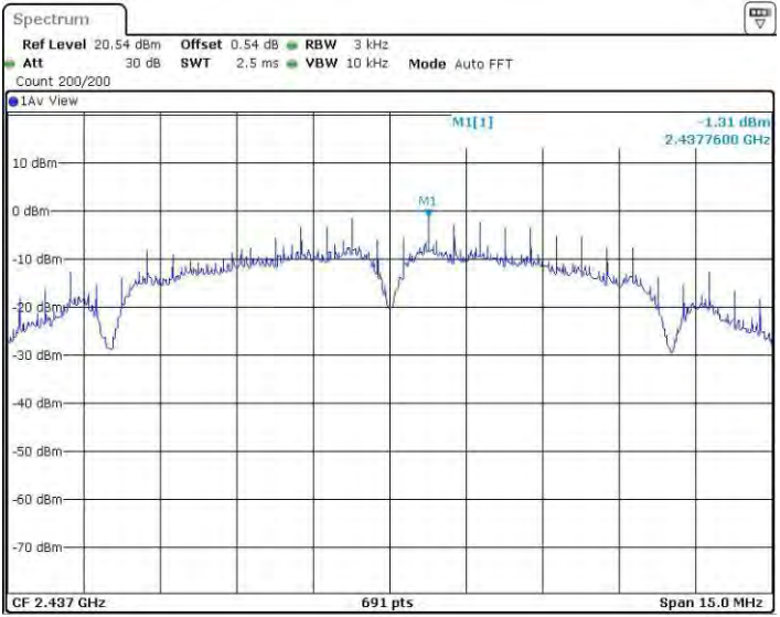
11BSISO_Ant1_2437
