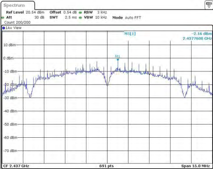
11BSISO_Ant4_2437
