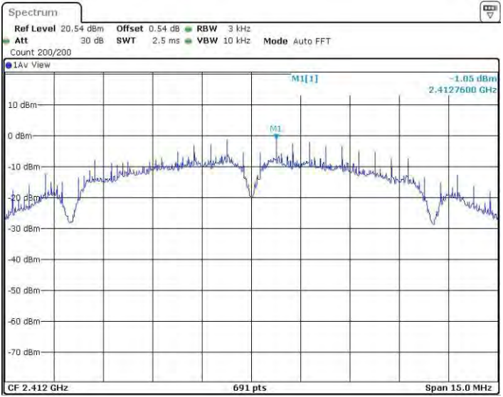
11BSISO_Ant2_2412
