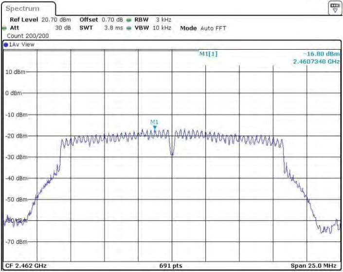
11GSISO_Ant3_2462
