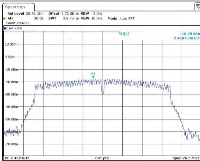
11N20SISO_Ant2_2462
