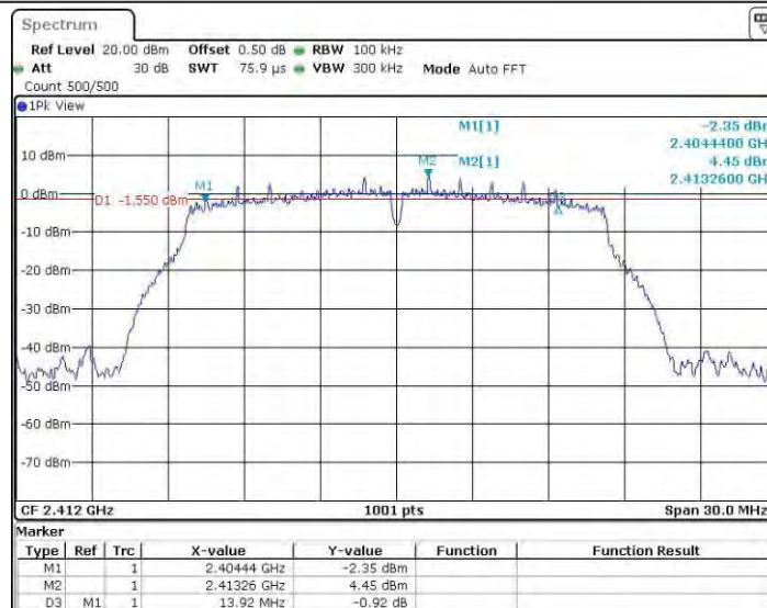
11GSISO_Ant3_2412
