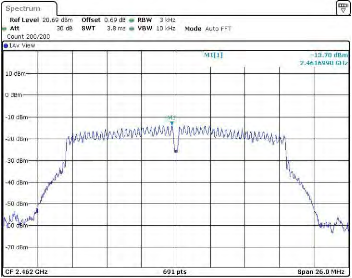
11G MIMO_Ant4_2462
