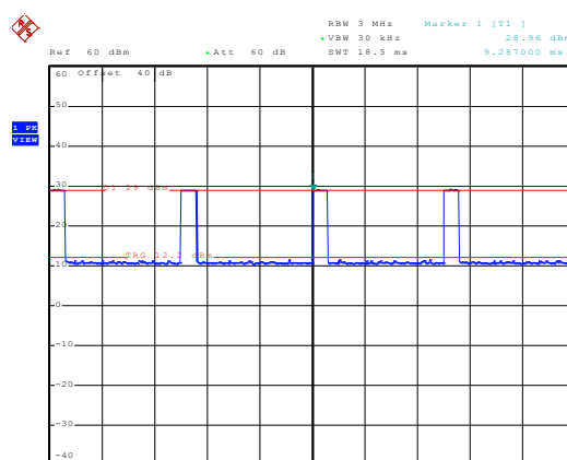
1880MHz - GSM
