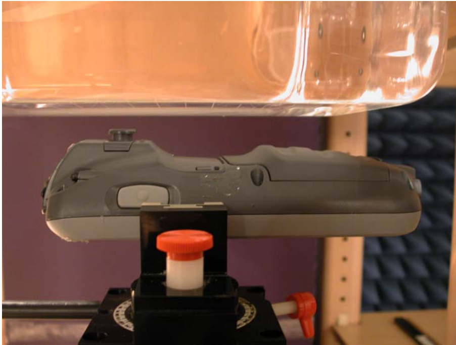
EUT Front (EUT distance 15mm)
