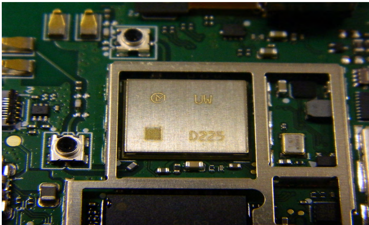
NFC Module
