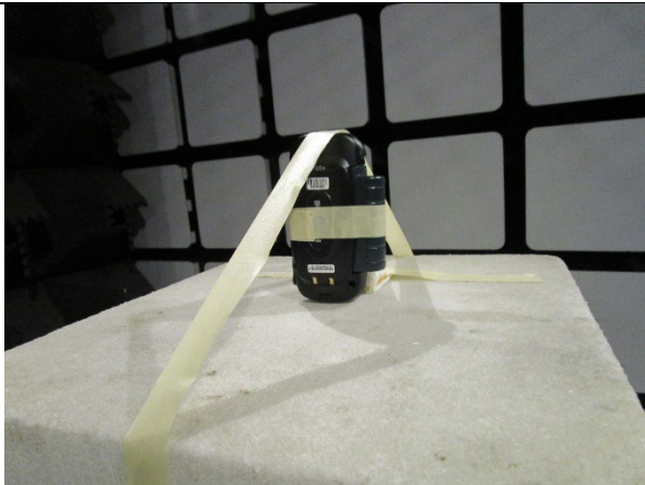
EUT Vertical
