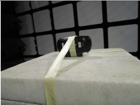
EUT Horizontal
