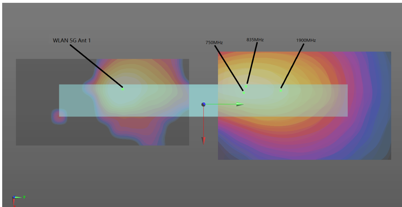
Edge 4 (0mm)+ WLAN5GHz(0mm)
