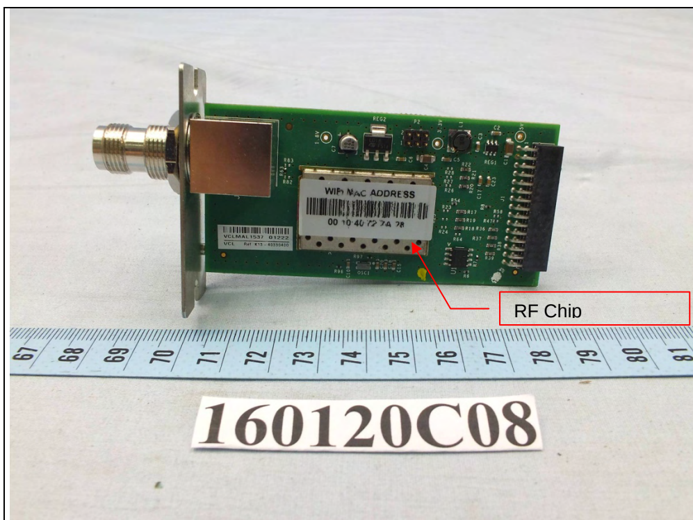
Wireless LAN & BT module
