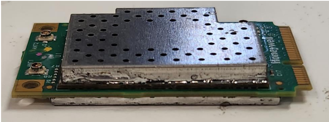
IM21-PRT RFID Module : Side View
