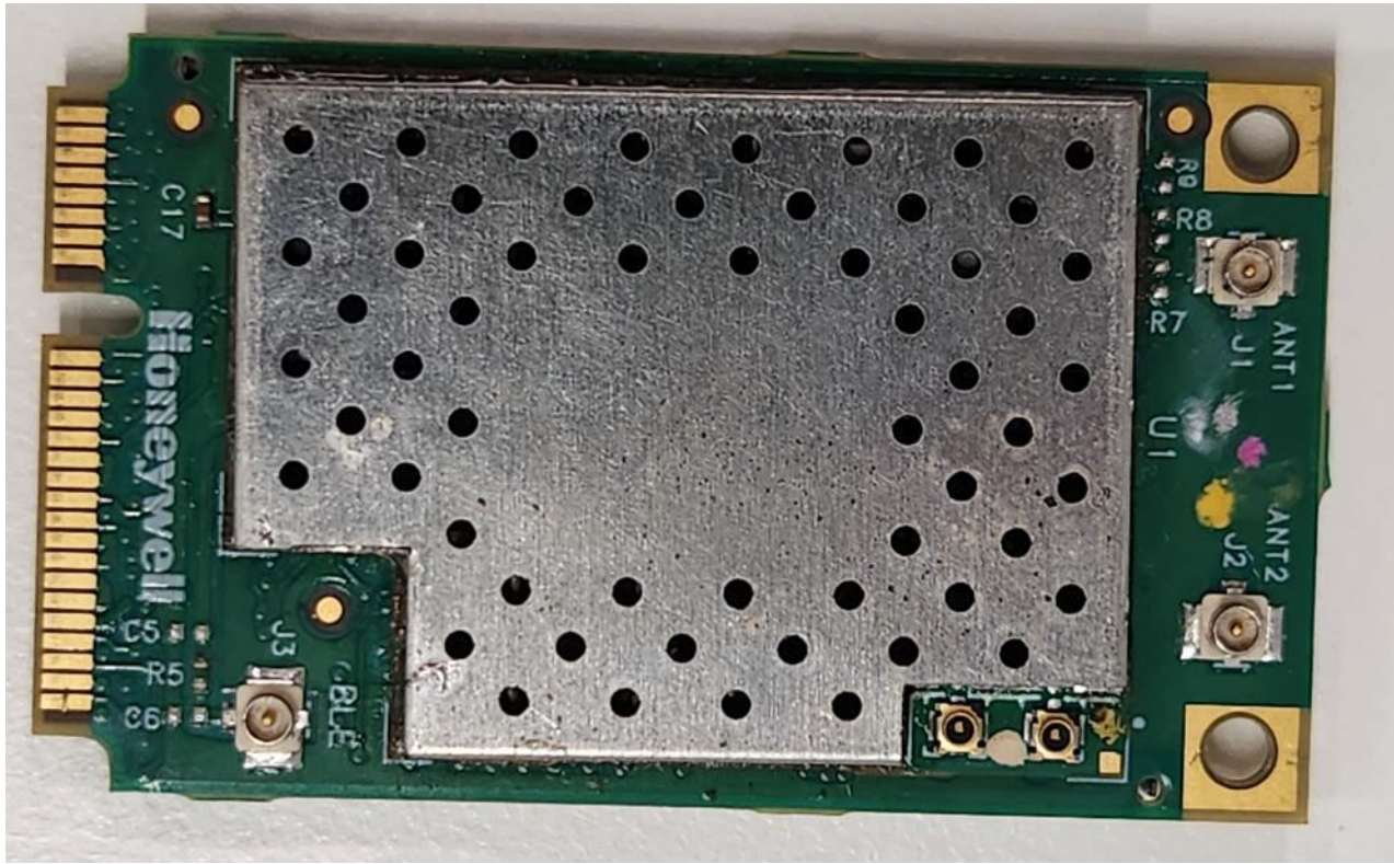
IM21-PRT RFID Module : Top View
