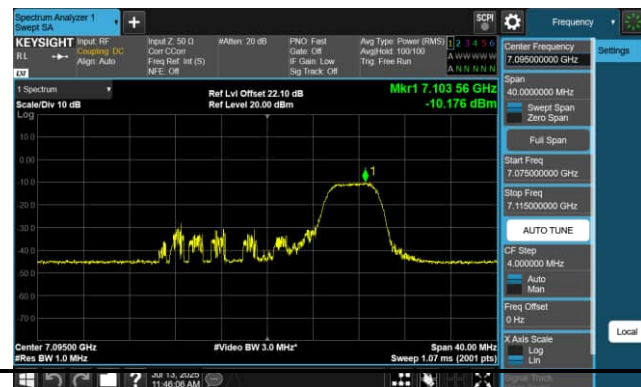
52 Tone_RU77_CH229 (7095MHz)
