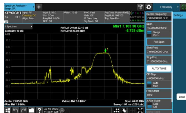
52 Tone_RU77_CH229 (7095MHz)
