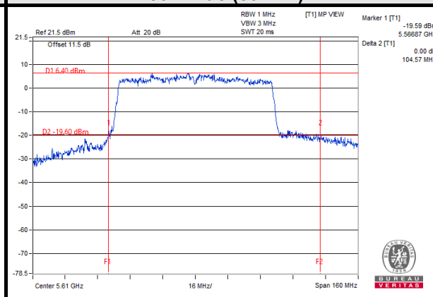
802.11ac (80MHz)
