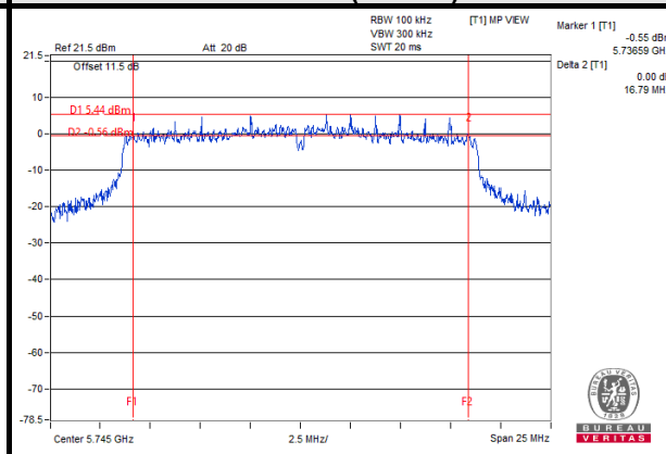
802.11ac (20MHz)
