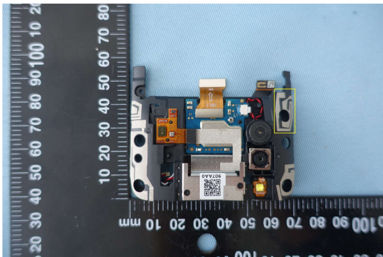
Ant 7 Wlan
