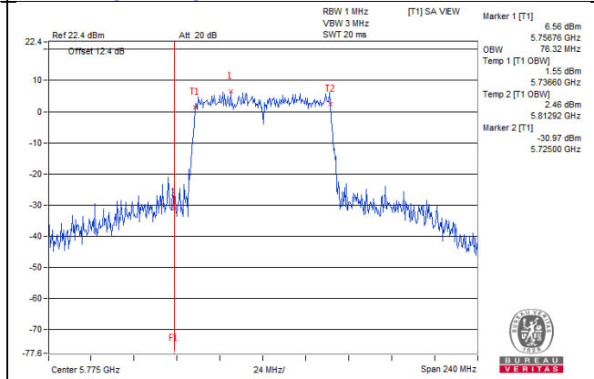
802.11ac(VHT80)_Chain1 / CH155
