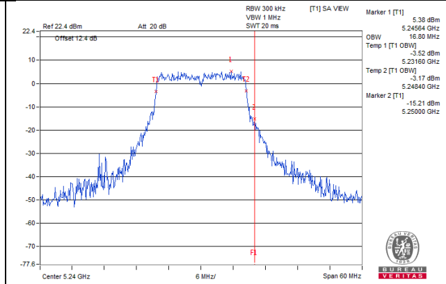
802.11ac(VHT20)_Chain1 / CH48
