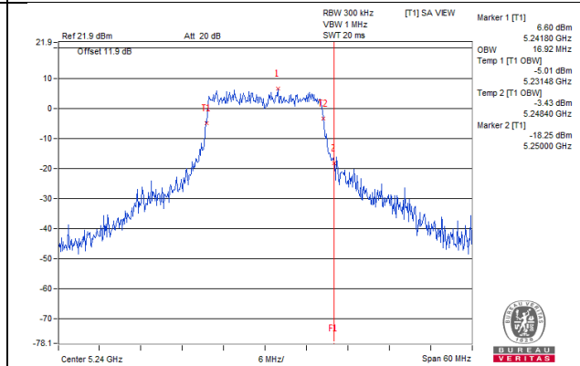
802.11ac(VHT20)_Chain1 / CH48
