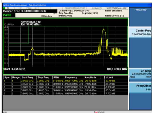
EDGE_5G_n77(N)_30KHz_P12-BPSK_20M_1RB@MAX_CH64666
