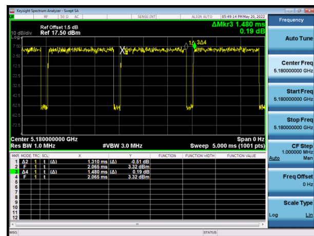
802.11ac(20MHz)
