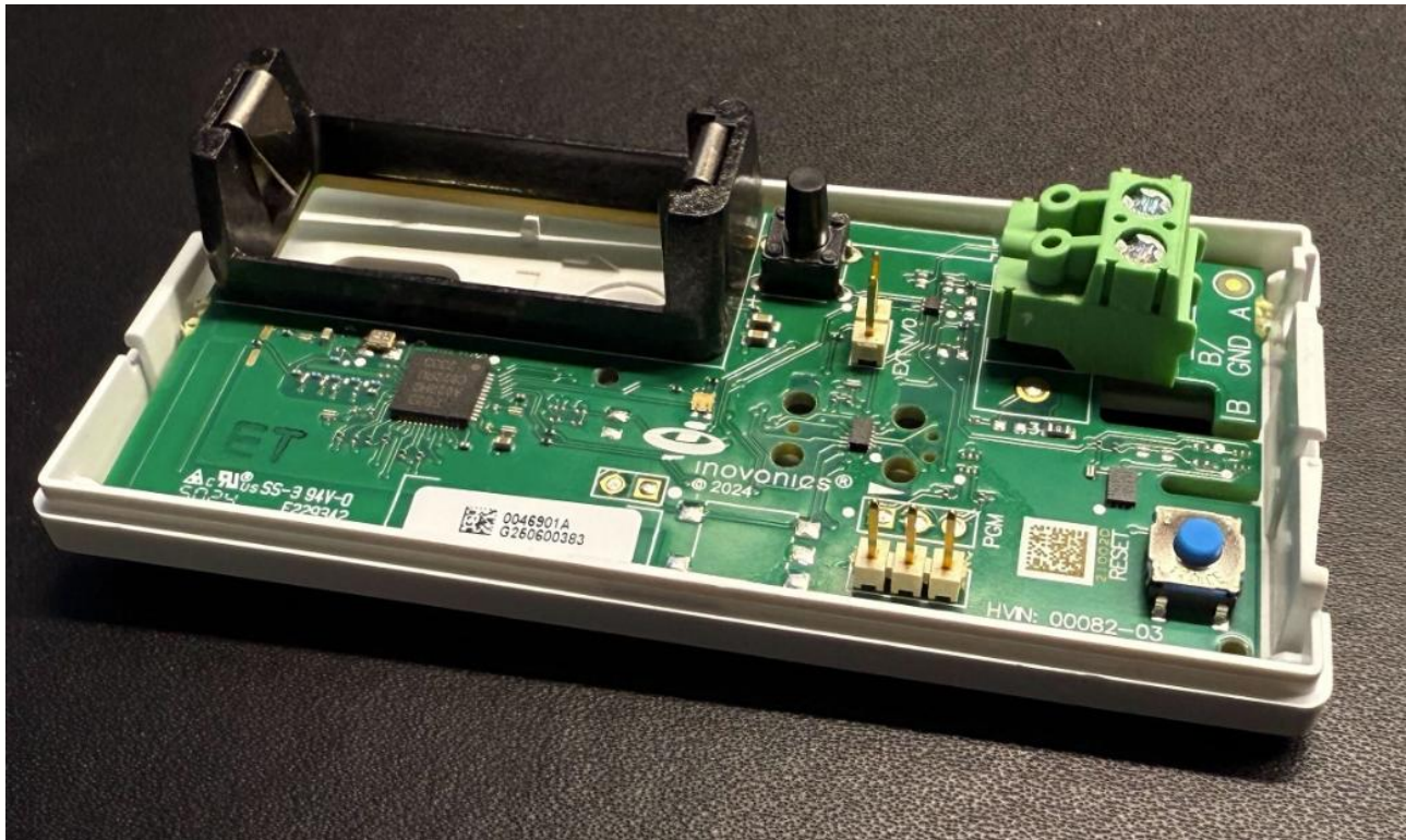
Top Main PCBA (EN1721)
