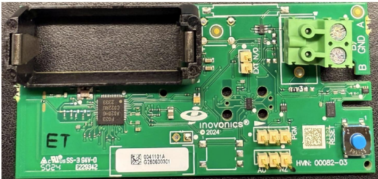
Top Main PCBA (EN1721)
