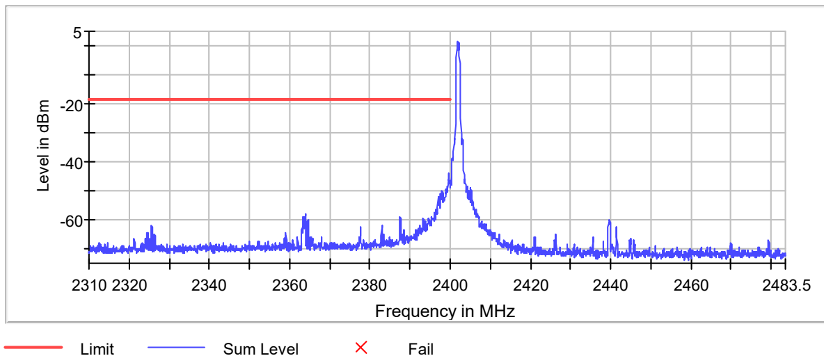
Band Edge
