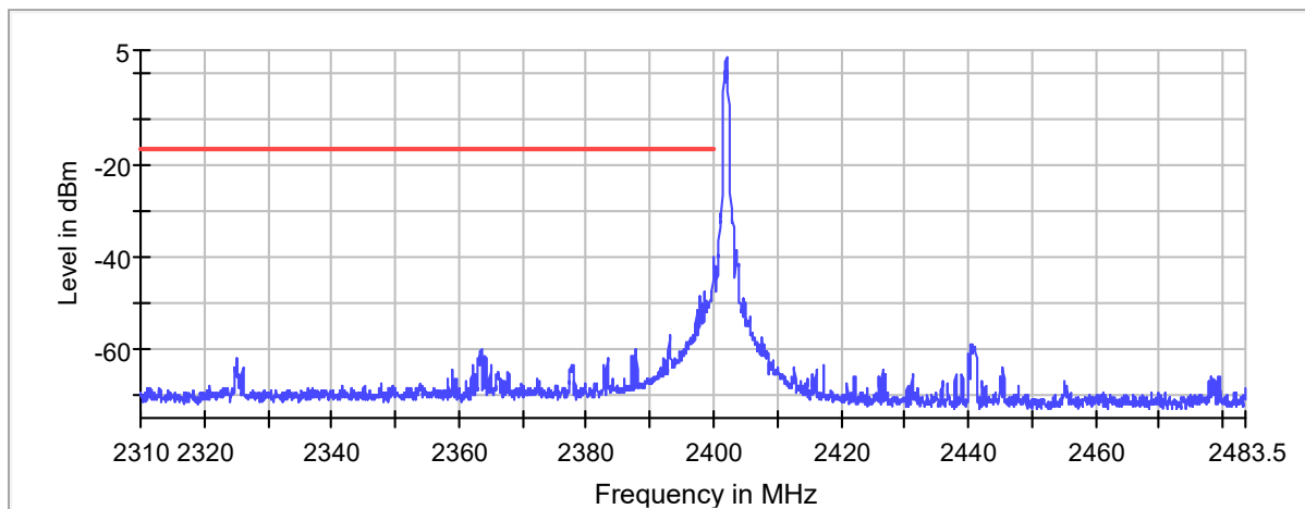
Band Edge
