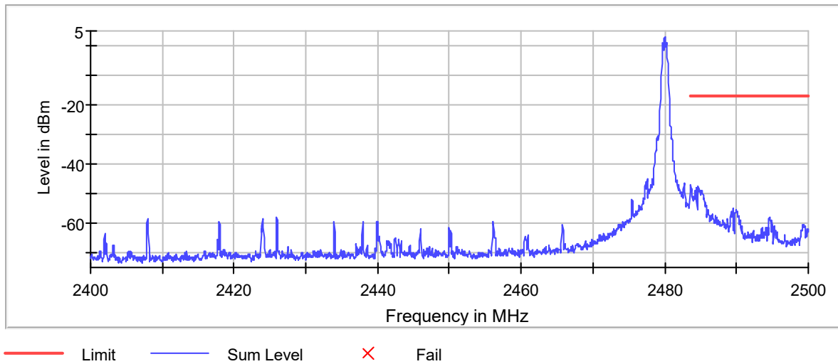
Band Edge
