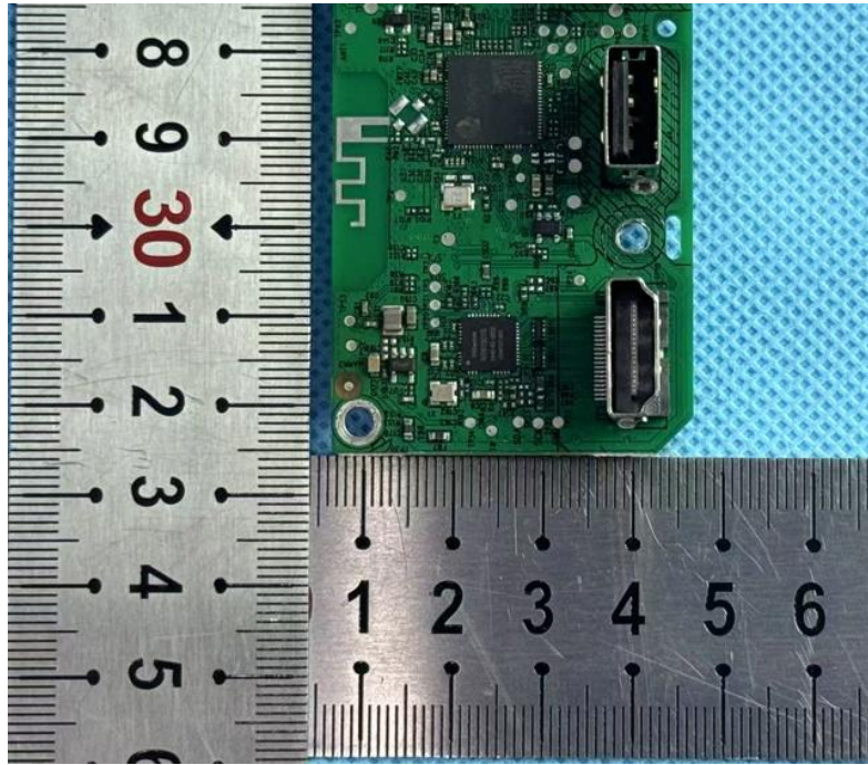
BT ANT
