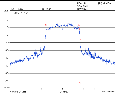
802.11ac(VHT80)_Chain2 / CH42
