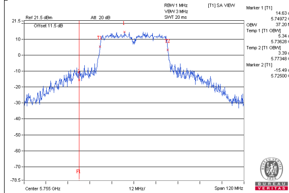
802.11ac(VHT40)_Chain3 / CH151
