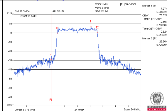
802.11ac(VHT80)_Chain3 / CH155
