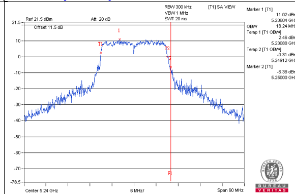
802.11ac(VHT20)_Chain3 / CH48
