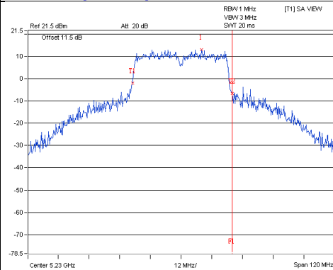
802.11ac(VHT40)_Chain2 / CH46
