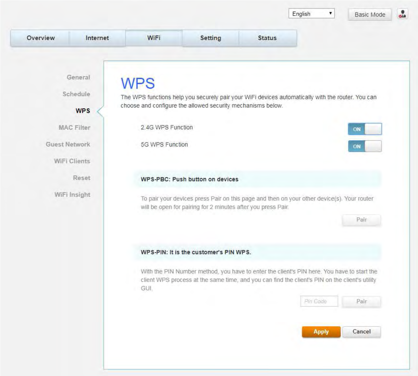
Fig.2-18 Wi-Fi\WPS
