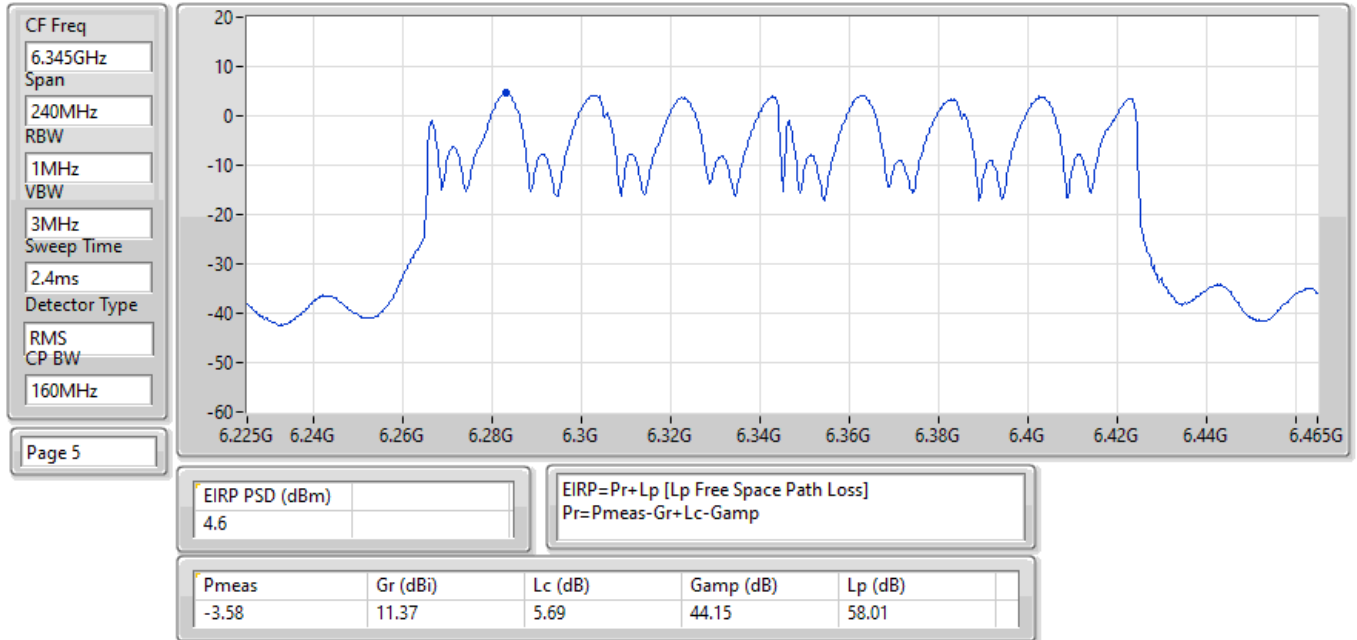
EIRP PSD;Band:6.2G;be160;BWch:160MHz;Nss:1,(M0);Nant:4;Ch:6345MHz;TX
