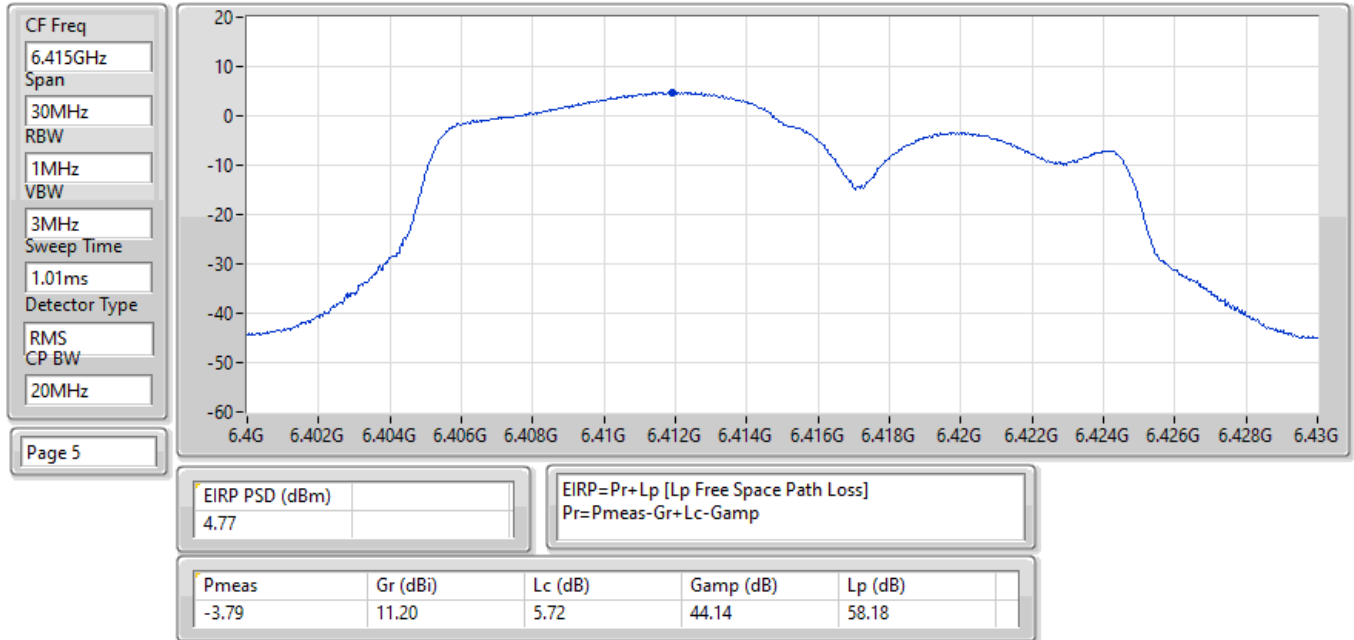
EIRP PSD;Band:6.2G;be20;BWch:20MHz;Nss:1,(M0);Nant:4;Ch:6415MHz;TX
