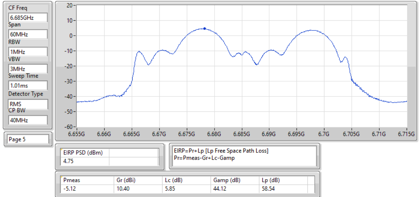
EIRP PSD;Band:6.7G;be40;BWch:40MHz;Nss:1,(M0);Nant:4;Ch:6685MHz;TX
