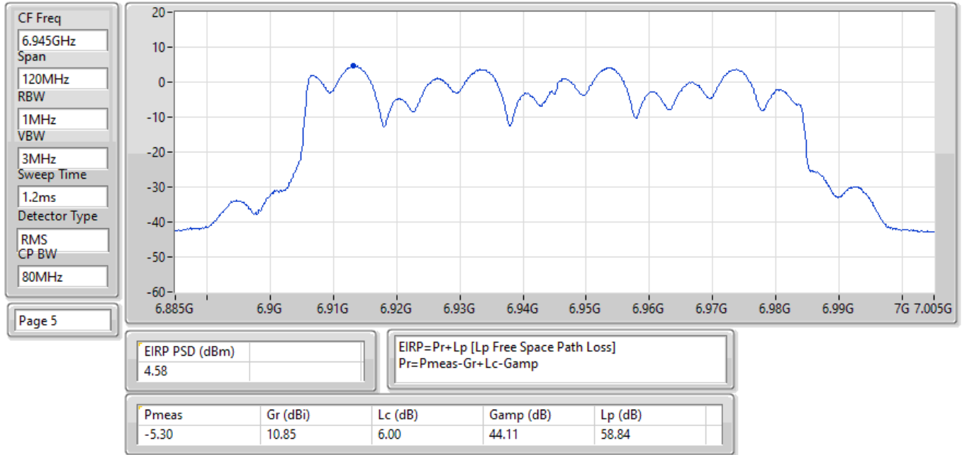
EIRP PSD;Band:7.0G;be80;BWch:80MHz;Nss:1,(M0);Nant:4;Ch:6945MHz;TX
