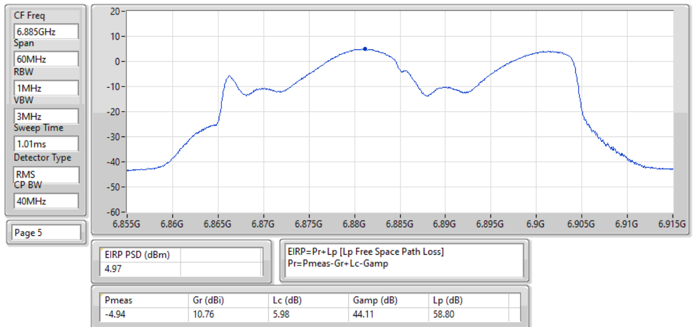
EIRP PSD;Band:6.7G;be40;BWch:40MHz;Nss:1,(M0);Nant:4;Ch:6885MHz;TX
