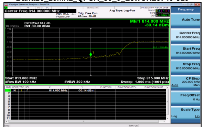
Band26 10MHz_QPSK_50_0_LowCH26740-819
