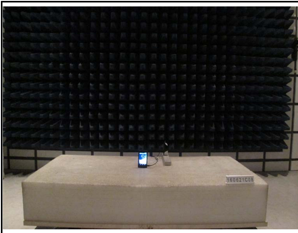
Z-Plane
