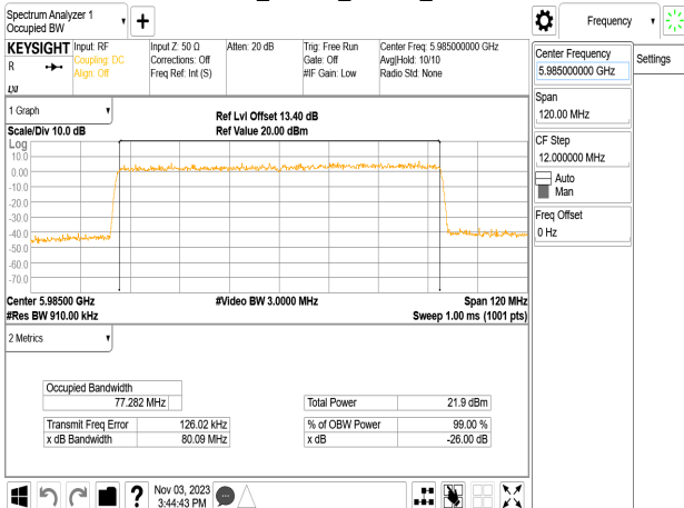
802.11be_80MHz_Chain0_5985MHz
