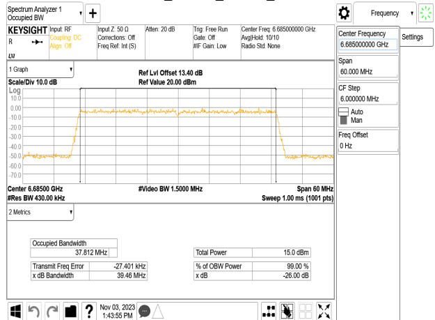
802.11be_40MHz_Chain0_6685MHz
