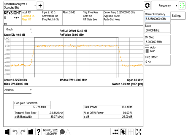
802.11be_40MHz_Chain2_6525MHz
