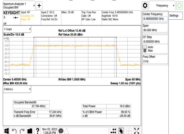
802.11be_40MHz_Chain3_6485MHz
