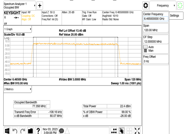
802.11be_80MHz_Chain0_6465MHz
