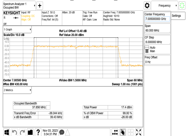
802.11be_40MHz_Chain2_7005MHz
