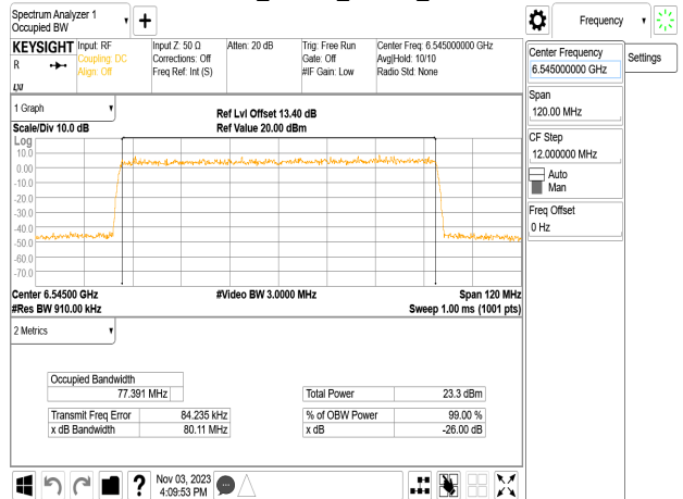
802.11be_80MHz_Chain1_6545MHz
