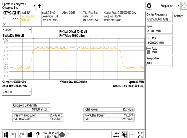
802.11be_20MHz_Chain3_6995MHz
