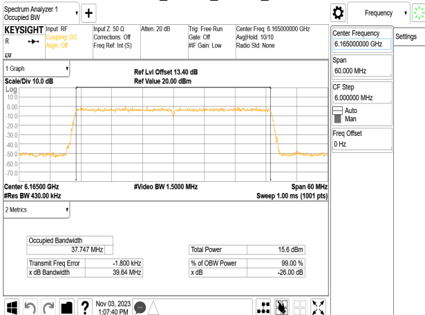
802.11be_40MHz_Chain3_6165MHz
