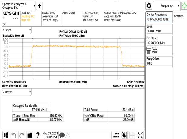
802.11be_80MHz_Chain1_6145MHz
