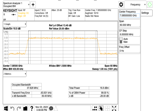
802.11be_40MHz_Chain1_7085MHz
