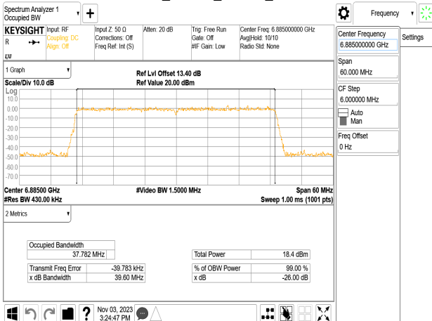
802.11be_40MHz_Chain1_6885MHz
