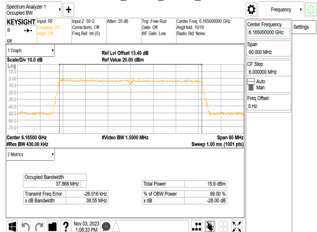
802.11be_40MHz_Chain0_6165MHz
