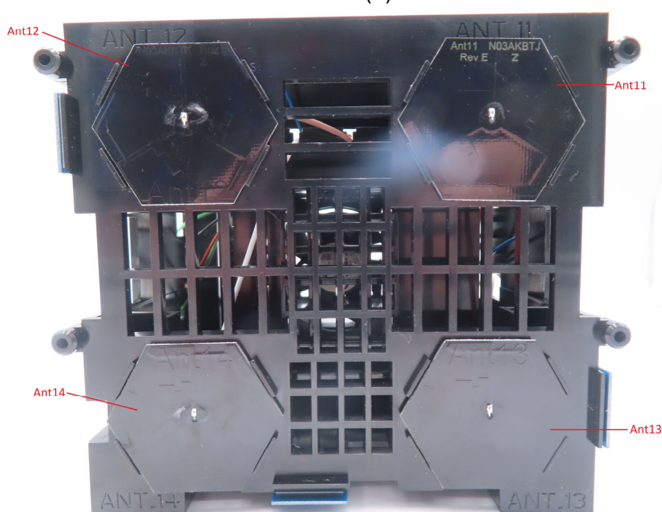
Antenna (1)
