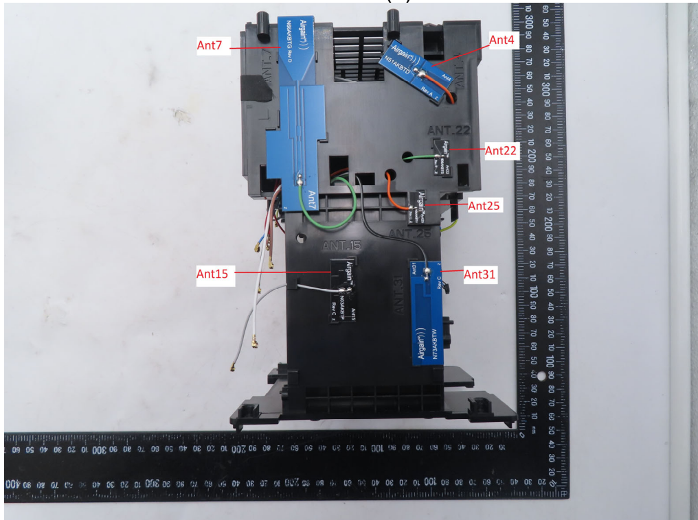
Antenna (3)
