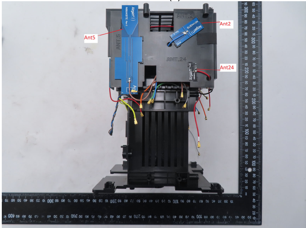
Antenna (5)
