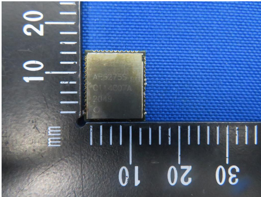
(3) Module Photo
