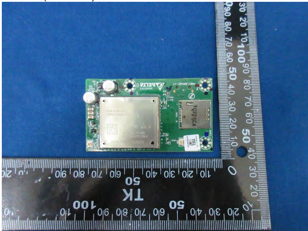
(30) EUT Photo (LTE Module)
