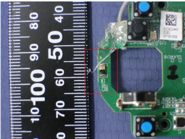
EUT (Antenna)
