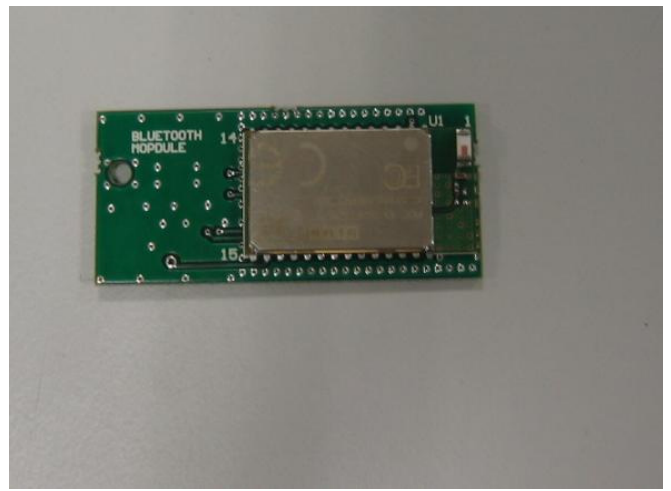
Bluetooth Module
