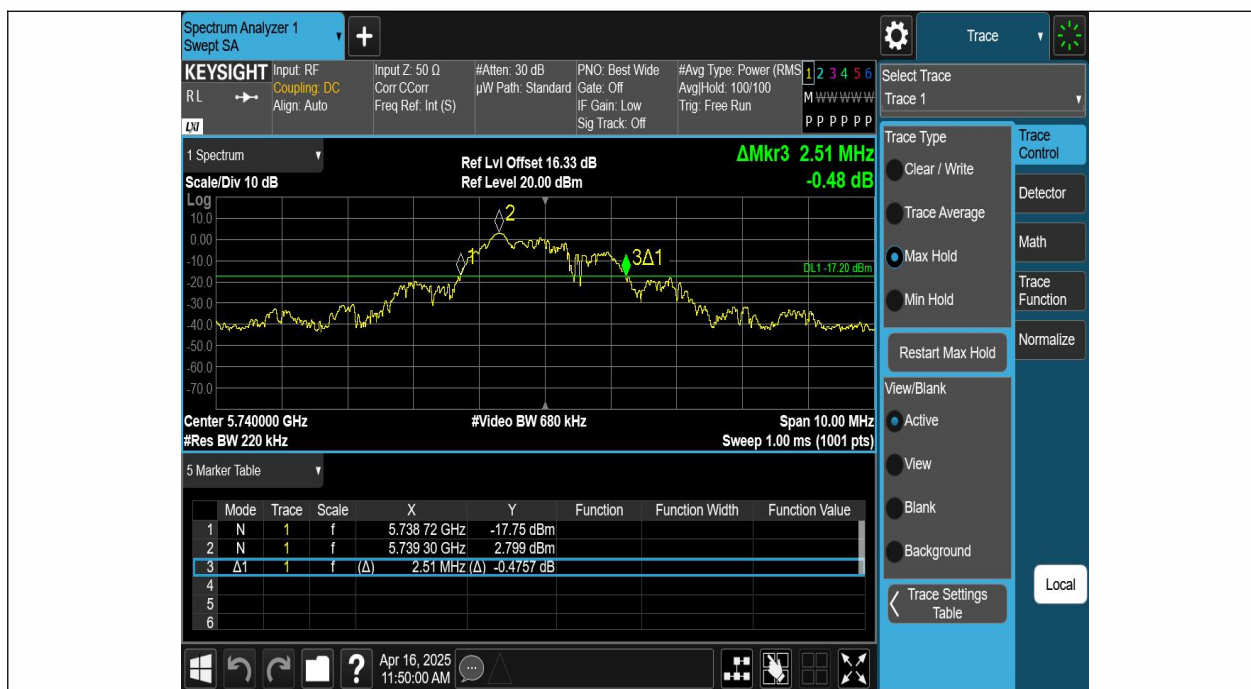
Ant1-5740
