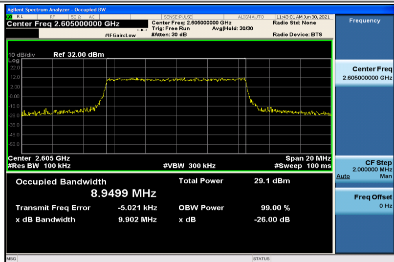
Band41-10MHz-QPSK-40740-50RB#0-8.9499
