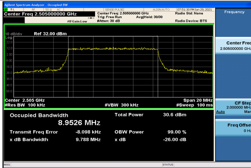
Band7-10MHz-QPSK-20800-50RB#0-8.9526
