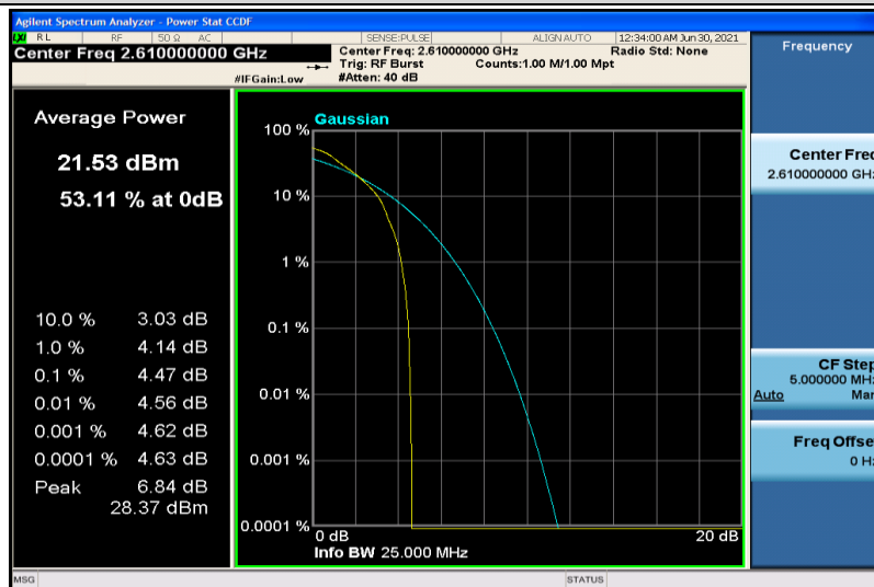
Band38-20MHz-QPSK-38150-1RB#0
