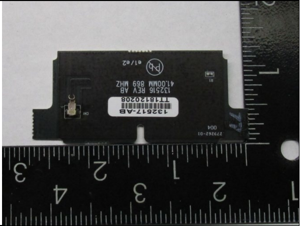
RFID Antenna
