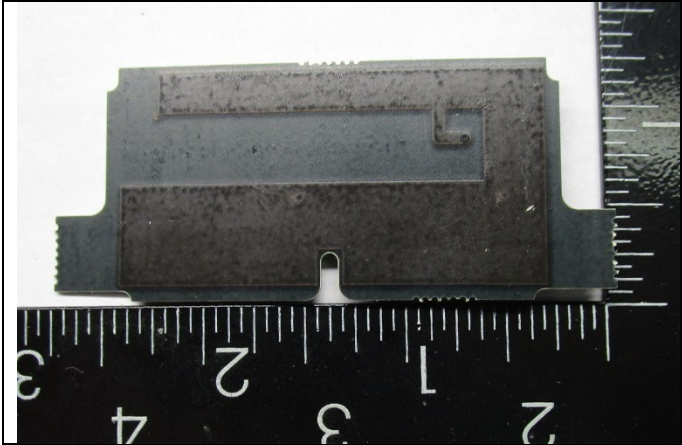
RFID Antenna
