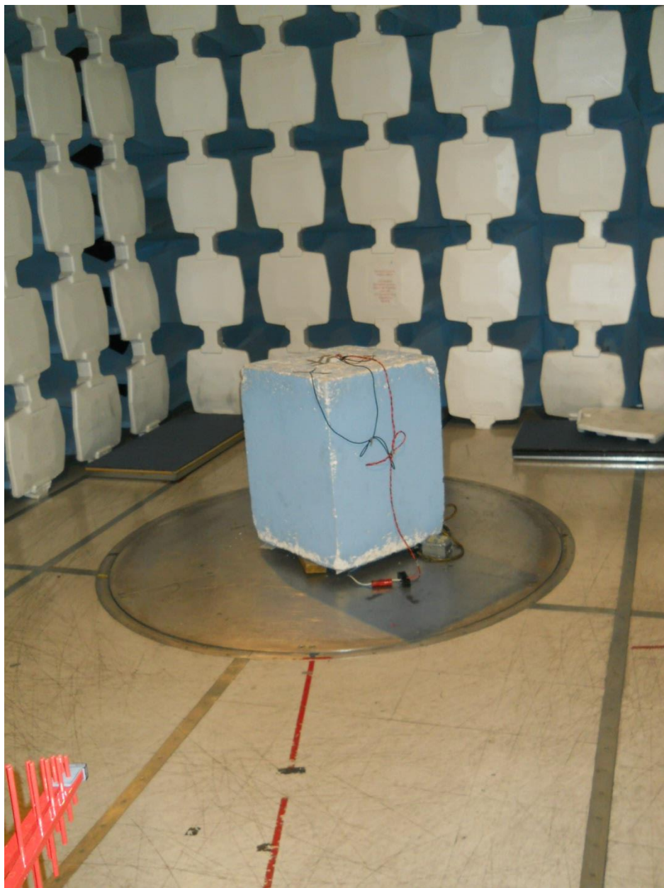
EMI 30 – 1000MHz
