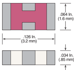
Case 18-2 (EIA 1206 / 3216)
