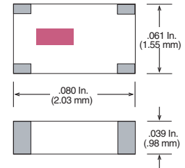
Case 15-4 (EIA 0805 / 1212)
