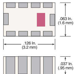
Case 18-4 (EIA 1206 / 3216)
