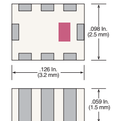
Case 41-2 (EIA 1210 / 3225)
