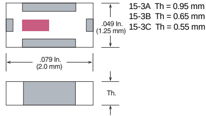
Case 15-3 (EIA 0805 / 1212)
