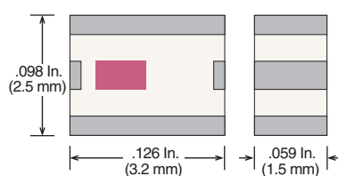
Case 41-1 (EIA 1210 / 3225)
