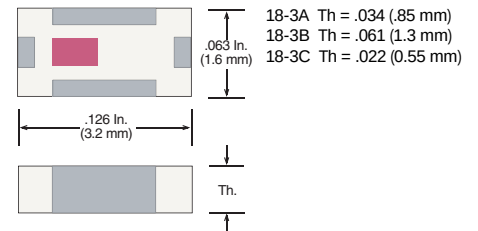
Case 18-3 (EIA 1206 / 3216)
