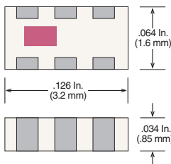
Case 18-1 (EIA 1206 / 3216)
