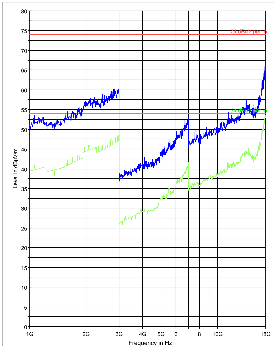
FCC 15 1-18GHz
