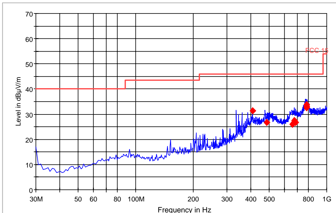
FCC 15 30-1000MHz
