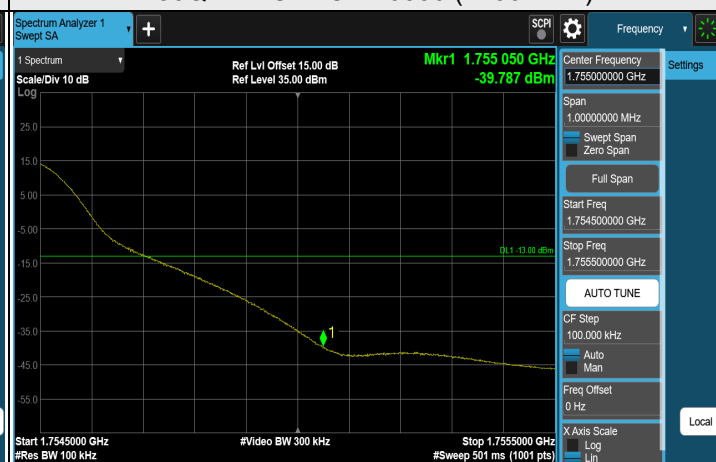
256QAM 1RB CH 20350 (1750 MHz)
