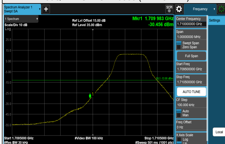
256QAM 1RB CH 19965 (1711.5 MHz)
