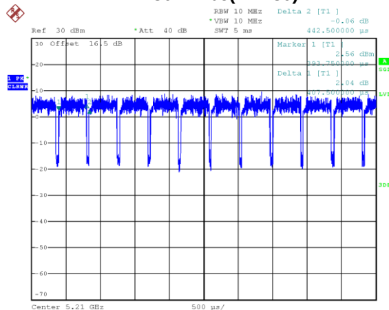
802.11be(EHT80)
