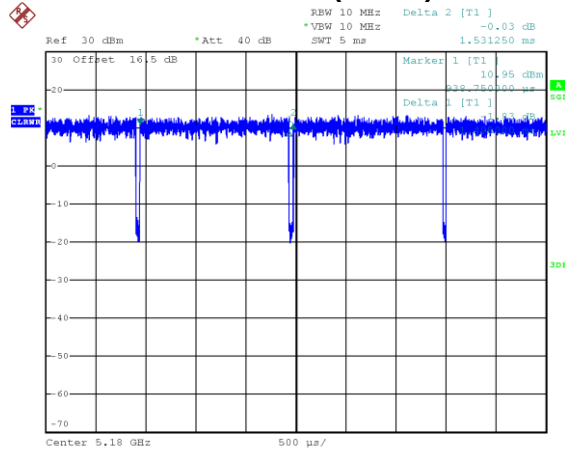
802.11be(EHT20)
