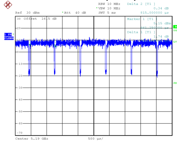
802.11be(EHT40)
