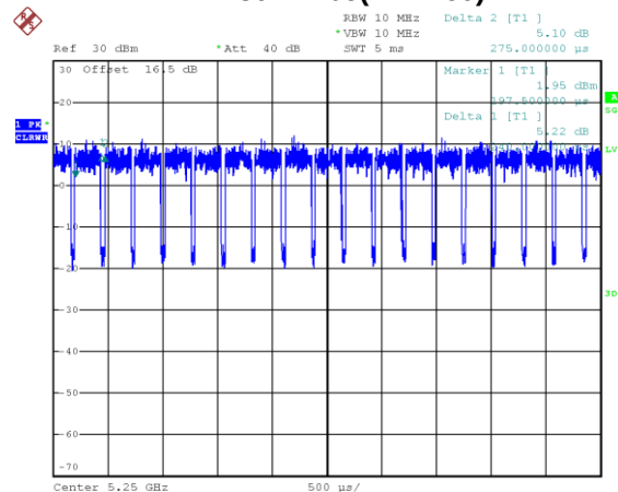
802.11be(EHT160)
