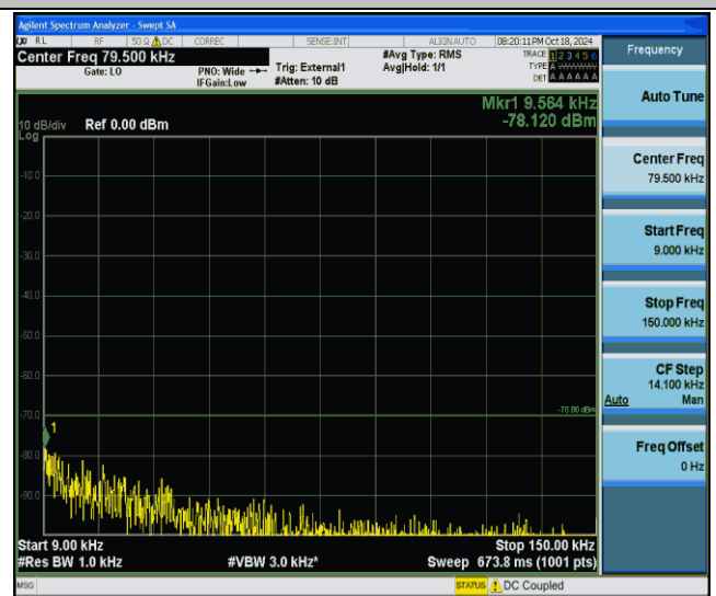
48-48-20MHz-20MHz-QPSK-QPSK-55891-56089-1RB#0-0RB#0- 0.009~0.15MHz-PASS
