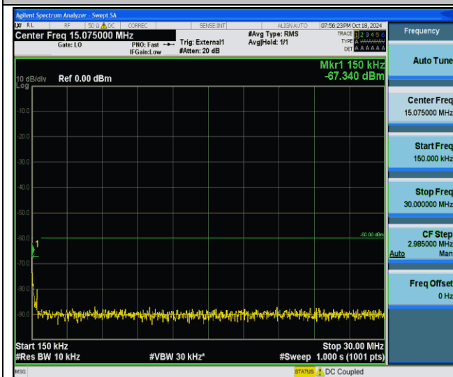
48-48-20MHz-20MHz-QPSK-QPSK-55891-56089-1RB#0-0RB#0- 0.15~30MHz-PASS
