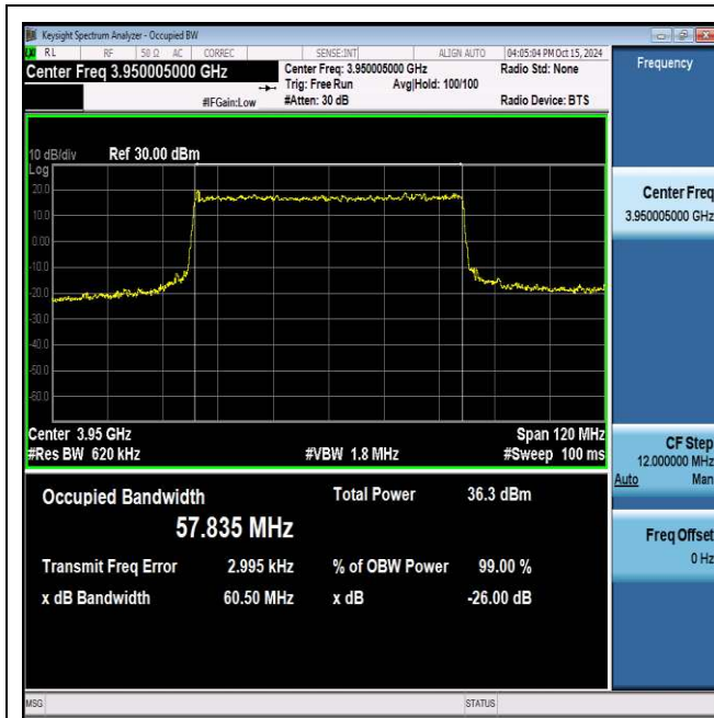
NTNV_N77-3700-3980_PC2_30_60_H_TID6_Ant1#1
