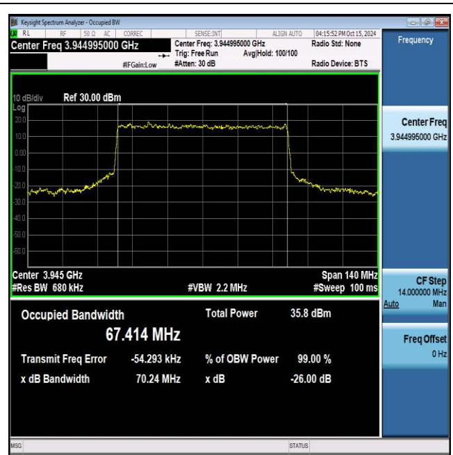
NTNV_N77-3700-3980_PC2_30_70_H_TID8_Ant1#1
