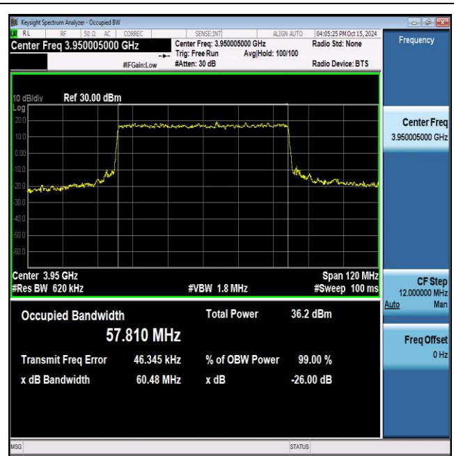
NTNV_N77-3700-3980_PC2_30_60_H_TID7_Ant1#1
