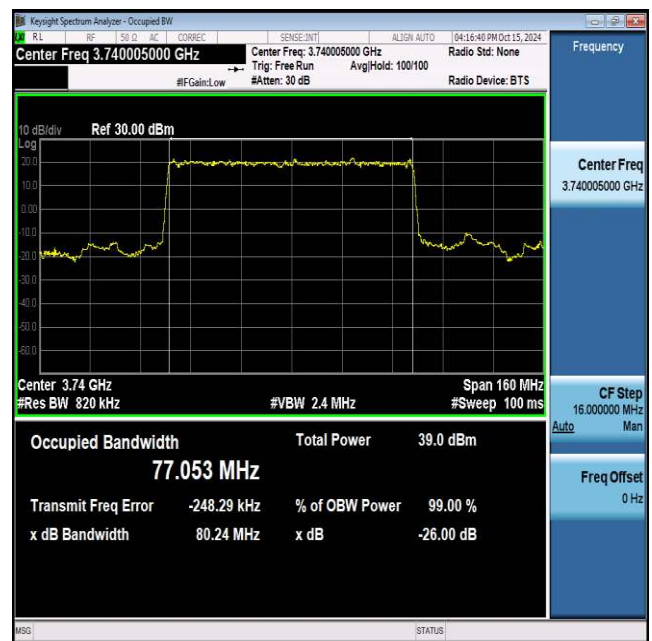
NTNV_N77-3700-3980_PC2_30_80_L_TID1_Ant1#1
