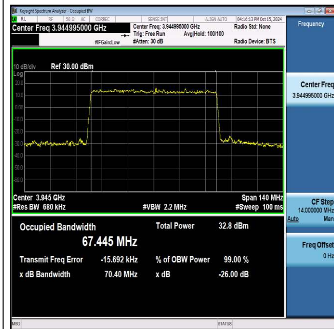
NTNV_N77-3700-3980_PC2_30_70_H_TID9_Ant1#1
