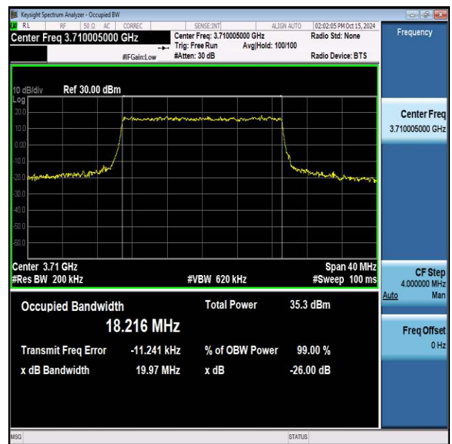
NTNV_N77-3700-3980_PC2_30_20_L_TID6_Ant1#1
