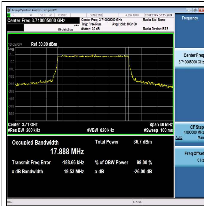
NTNV_N77-3700-3980_PC2_30_20_L_TID3_Ant1#1
