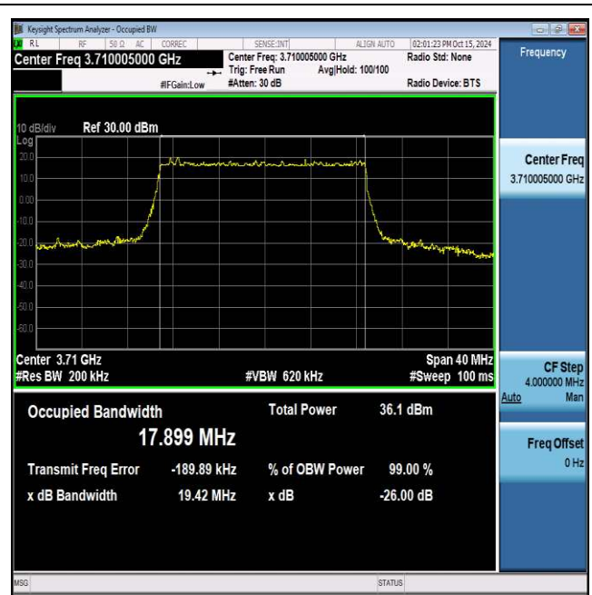
NTNV_N77-3700-3980_PC2_30_20_L_TID4_Ant1#1
