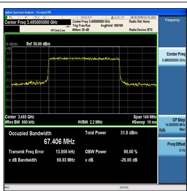
NTNV_N77-3450-3550_PC2_30_70_L_TID6_Ant1#1
