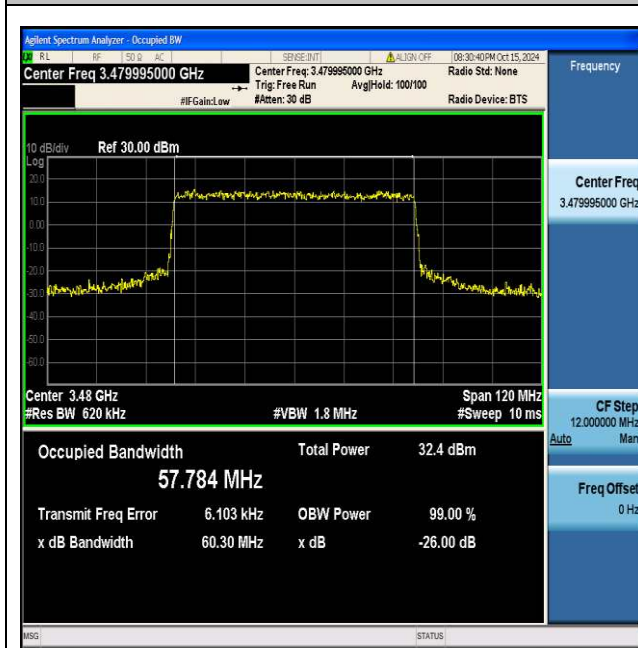
NTVN_N77-3450-3550_PC2_30_60_L_TID3_Ant1#1
