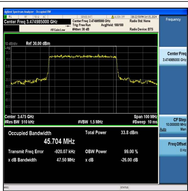
NTNV_N77-3450-3550_PC2_30_50_L_TID2_Ant1#1
