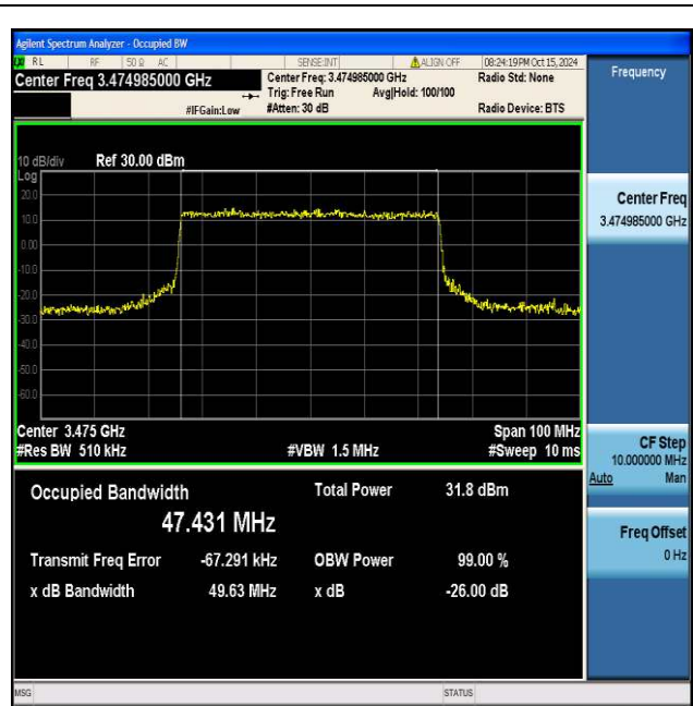
NTNV_N77-3450-3550_PC2_30_50_L_TID6_Ant1#1
