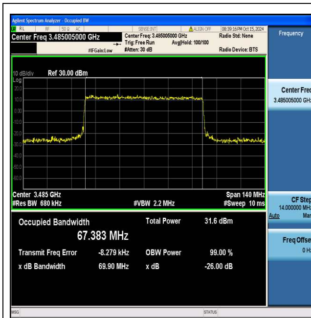
NTNV_N77-3450-3550_PC2_30_70_L_TID5_Ant1#1
