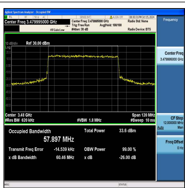
NTVN_N77-3450-3550_PC2_30_60_L_TID2_Ant1#1
