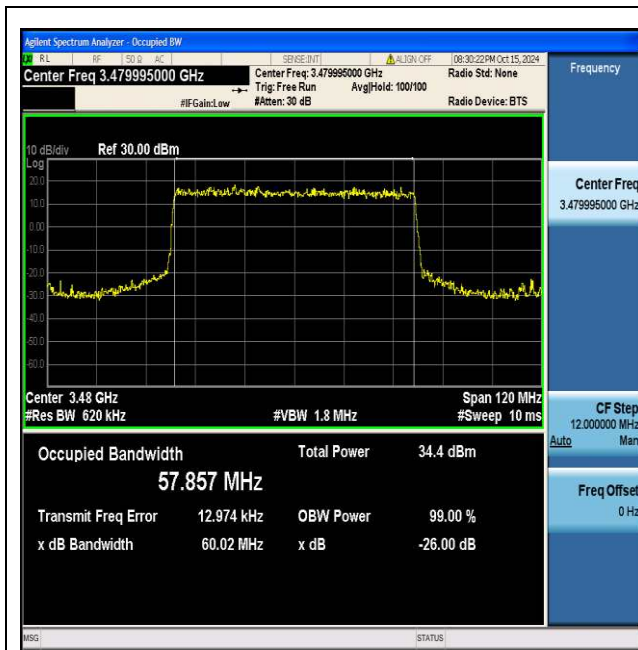
NTVN_N77-3450-3550_PC2_30_60_L_TID1_Ant1#1
