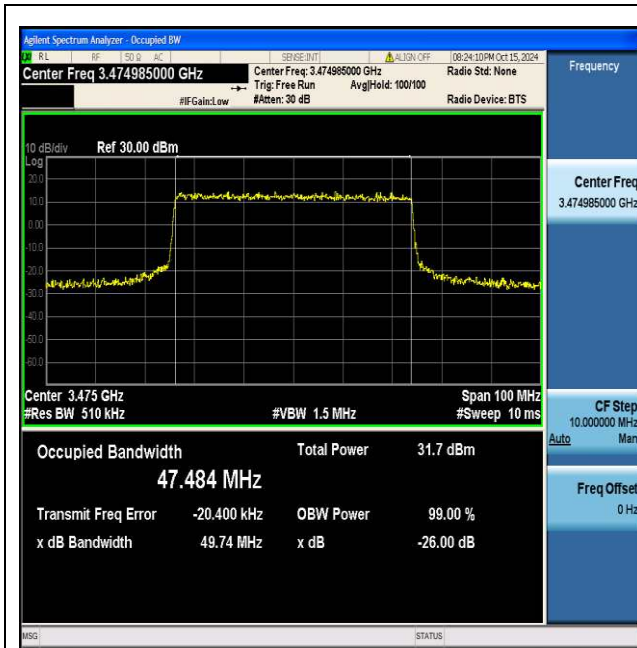
NTNV_N77-3450-3550_PC2_30_50_L_TID5_Ant1#1
