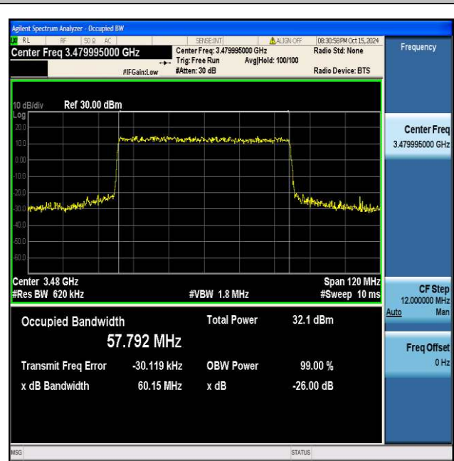
NTVN_N77-3450-3550_PC2_30_60_L_TID4_Ant1#1
