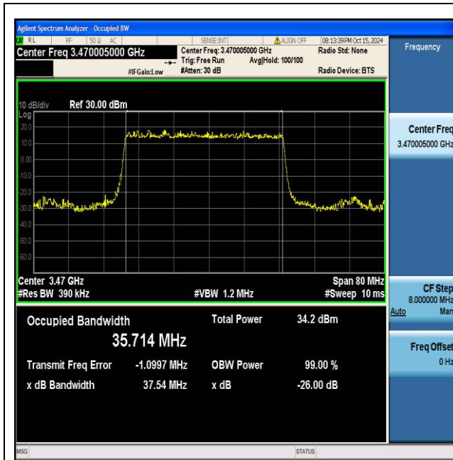
NTNV_N77-3450-3550_PC2_30_40_L_TID1_Ant1#1
