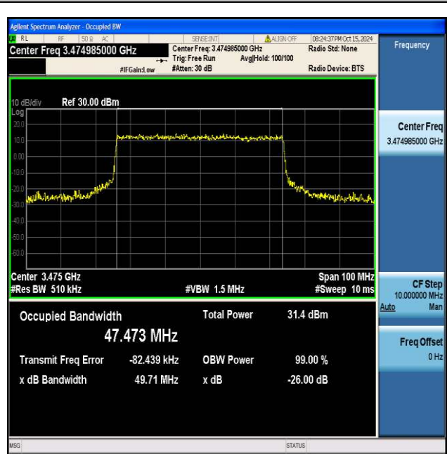
NTNV_N77-3450-3550_PC2_30_50_L_TID8_Ant1#1
