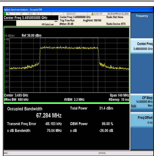
NTNV_N77-3450-3550_PC2_30_70_L_TID8_Ant1#1
