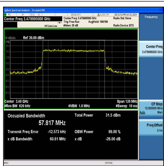
NTNV_N77-3450-3550_PC2_30_60_L_TID6_Ant1#1
