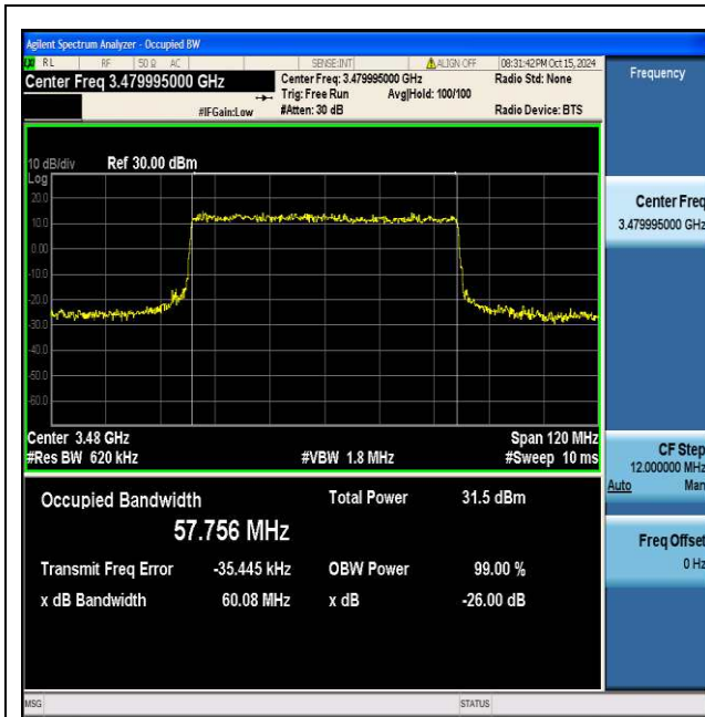
NTNV_N77-3450-3550_PC2_30_60_L_TID5_Ant1#1
