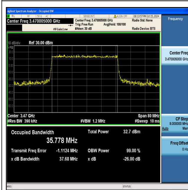
NTNV_N77-3450-3550_PC2_30_40_L_TID3_Ant1#1
